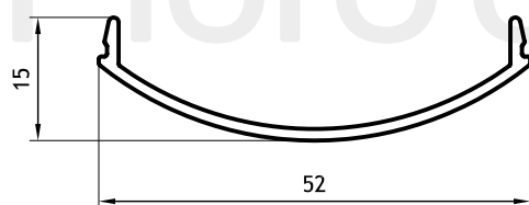
Tapa pasamanos 0,255 kg/m 9202 Barras de 6,20m
