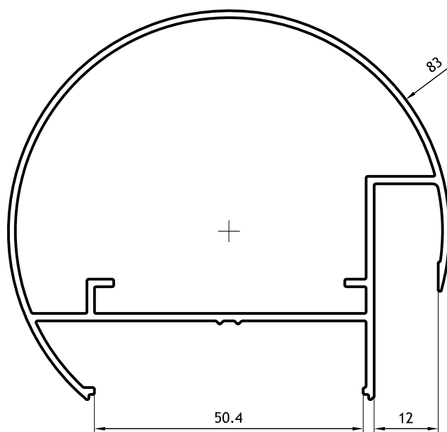
Pasamanos redondo 1,160 kg/m 9200 Barras de 6,20m
