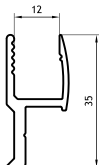
Soporte Vidrio 0,410 kg/m 09204 Barras de 6.20m
