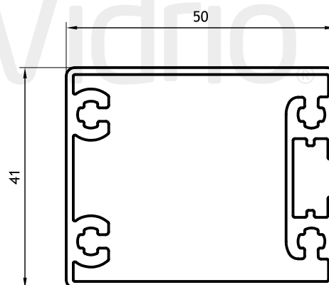
Columna Baranda Balcon 1,000 kg/m 09203 Barras de 6.05m
