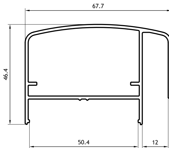
Pasamanos rectangular 0,930 kg/m 9201 Barras de 6,20m
