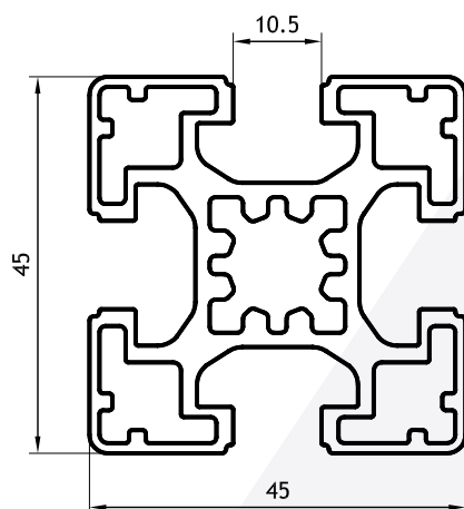
Parante Cuadrado Pesado 1,680 Kg/m 05062 (Barras de 6.05m)
