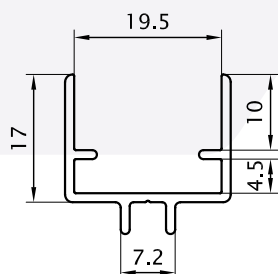
Soporte para panel 18mm 0,220 Kg/m 06208 (Barras de 6.05m)
