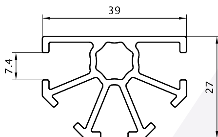
Parante 180° 0,730 Kg/m 06205 (Barras de 6.05m)
