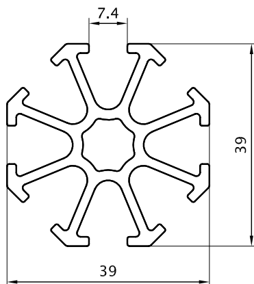
Parante 360° 1,006 Kg/m 06201 (Barras de 6.05m)
