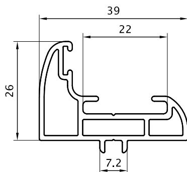
Marco para código 6210 0,540 Kg/m 06211 (Barras de 6.05m)
