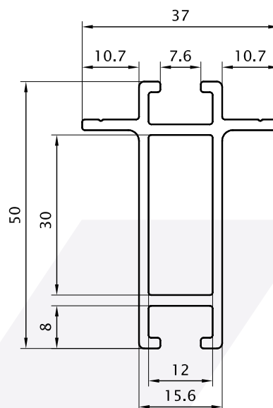
Travesaño con doble ala 0,780 Kg/m 06212 (Barras de 6.05m)
