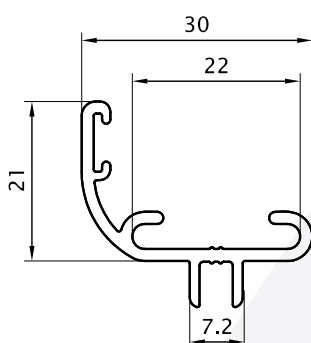
Marco Mini para Hoja de Abrir 0,330 Kg/m 06209 (Barras de 6.05m)
