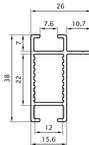
Travesaño con ala liviano 0,451 Kg/m 06207 (Barras de 6.05m)
