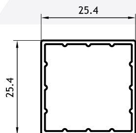
Parante Tubular 25mm 0,284 Kg/m 06215 (Barras de 6.05m)
