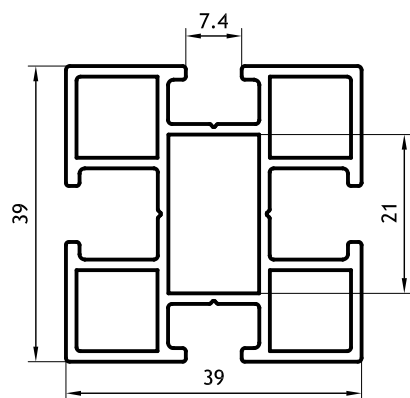
Parante Cuadrado Liviano 1,000 Kg/m 06210 (Barras de 6.05m)
