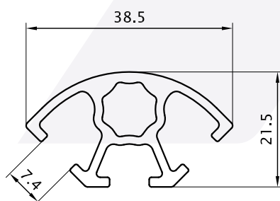
Parante 90° 0,540 Kg/m 06206 (Barras de 6.05m)
