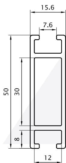
Travesaño 50mm 0,661Kg/m 06213 (Barras de 6.05m)
