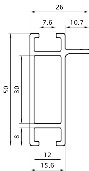
Travesaño con ala 0,721 Kg/m 06200 (Barras de 6.05m)
