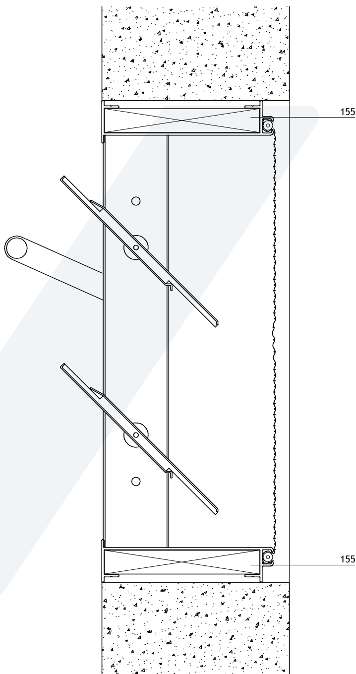
CORTE 1-2
