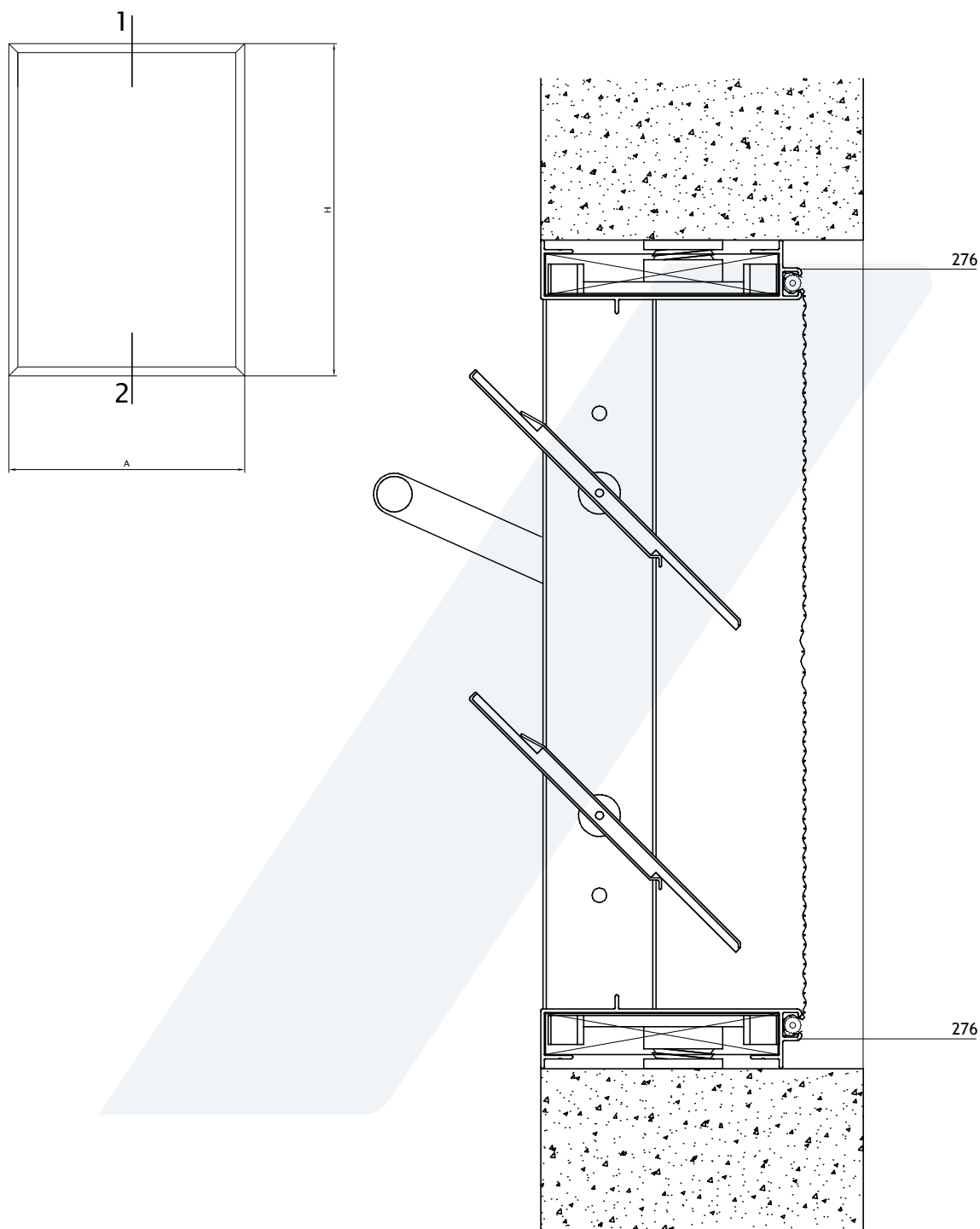
CORTE 1-2
