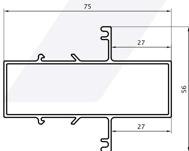
Travesaño 0,923 kg/m 00114 (Barras de 6.05m) 4 Barras por Paquete
