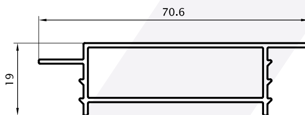
Premarco 0,494 Kg/m 00147 (Barras de 6.05m) 10 Barras por Paquete
