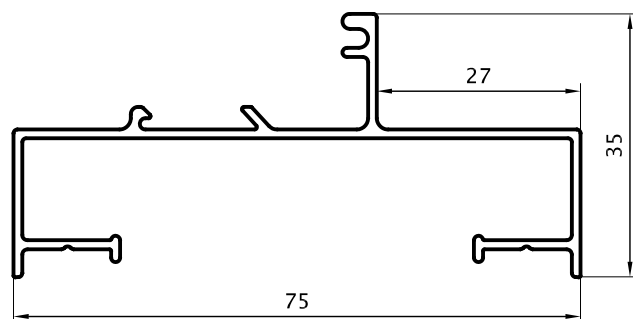
Marco Paño Fijo 75mm 0,563 kg/m 00107 (Barras de 6,20m) 8 Barras por Paquete
