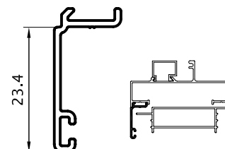
Tapajuntas 0,148 Kg/m 09013 (Barras de 6.05m) 18 Barras por Paquete
