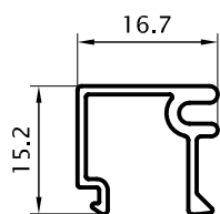
Contravidrio 0,172 kg/m 00108 (Barras de 6.05m) 30 Barras por Paquete
