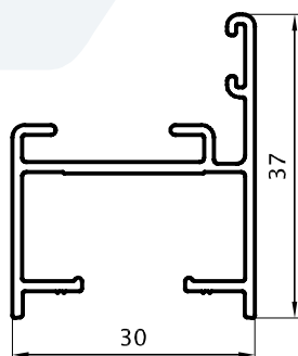
Marco Angosto 30mm 0,408 kg/m 00165 (Barras de 6.05m) 12 Barras por Paquete
