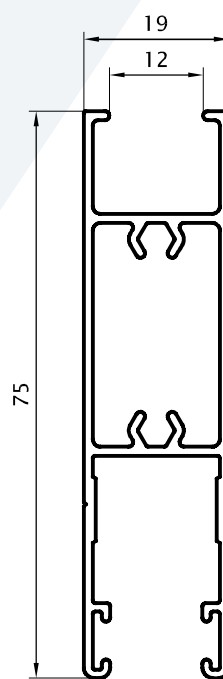
Travesaño 75mm 0,750 kg/m 00113 (Barras de 6.05m)
