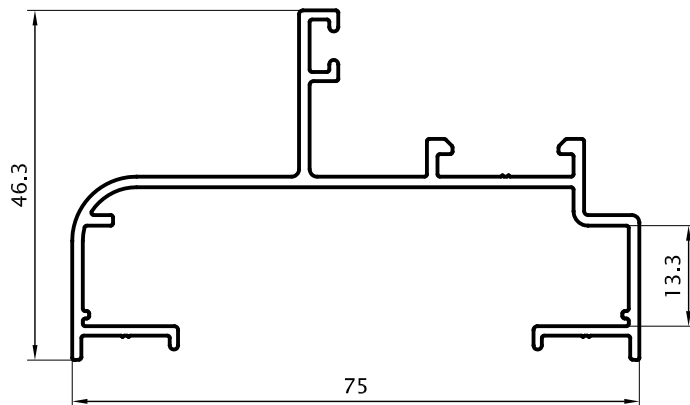
Marco Puerta y Ventana de Abrir 0,720 kg/m 02851 Barras de 6.05m 8 Barras por Paquete
