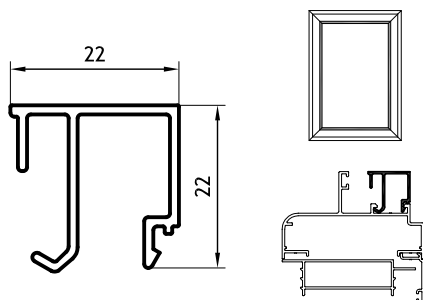
Contravidrio Recto Alojamiento 17mm 0,258 Kg/m 03209 Barras de 6.05m 20 Barras por Paquete
