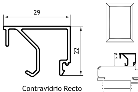
S Contravidrio Recto 0,298 Kg/m 03210 Barras de 6.05m 20 Barras por Paquete
