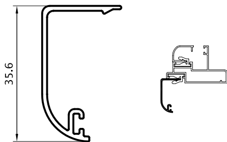
Tapajunta Enclipable 0,250 kg/m 02826 (Barras de 6.05m) 18 Barras por Paquete
