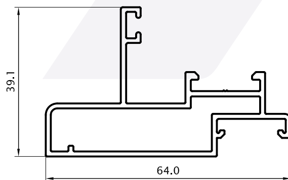
Marco Puerta y Ventana de Abrir Tubular 0,770 kg/m 02825 Barras de 6.05m 8 Barras por Paquete
