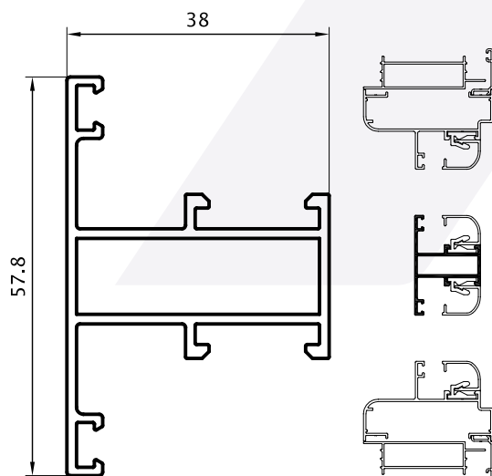
Travesaño para Paño Fijo Recto 0.720 kg/m 03203 (Barras de 6.05m)
