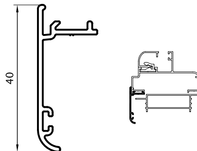
Tapajuntas 0,251 kg/m 09011 (Barras de 6.05m)
