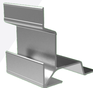
70604 Escuadra 13mm Pesada para Perfil 147 (45,5mm) x 100 unidades
