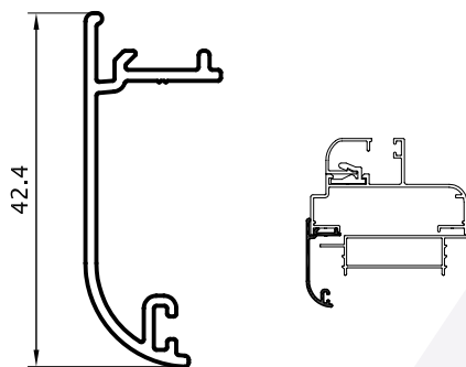
Tapajuntas 0,312 kg/m 09012 (Barras de 6.05m)
