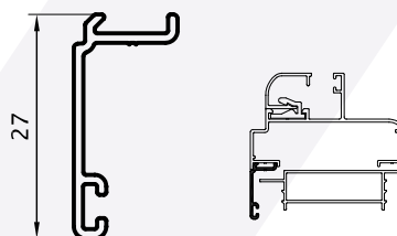
Tapajuntas 0,148 kg/m 09013 (Barras de 6.05m)
