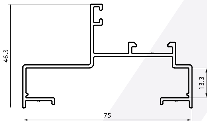
Marco Recto Puerta y Ventana de Abrir 0,724 kg/m 02855 Barras de 6.05m 8 Barras por Paquete
