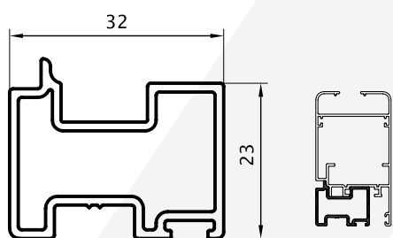
Zócalo Puerta de Abrir 0,375 kg/m 02852 Barras de 6.05m 10 Barras por Paquete
