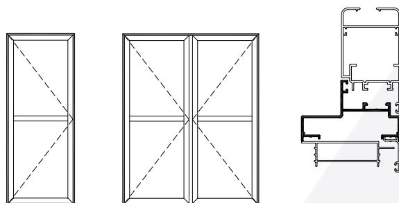
Marco Puerta y Ventana de Abrir 0,720 kg/m 02851 Barras de 6.05m 8 Barras por Paquete
