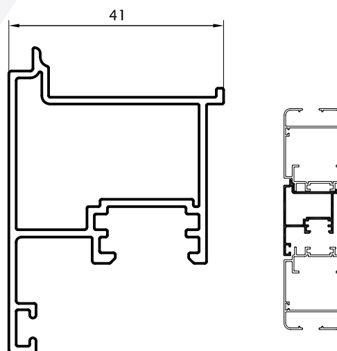
Encuentro Hojas de Abrir 0,754 kg/m 02853 Barras de 6.05m 6 Barras por Paquete
