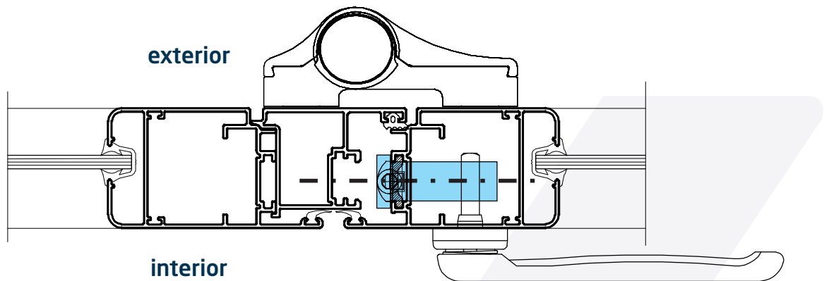
Apertura desde el interior
