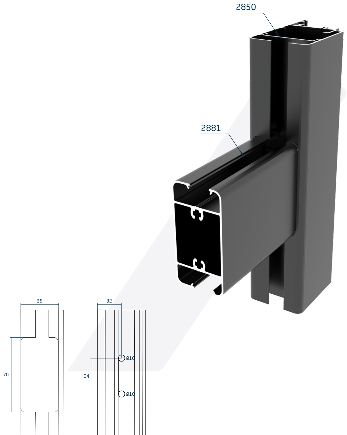
Mecanizado para travesaño Cód. 2850
