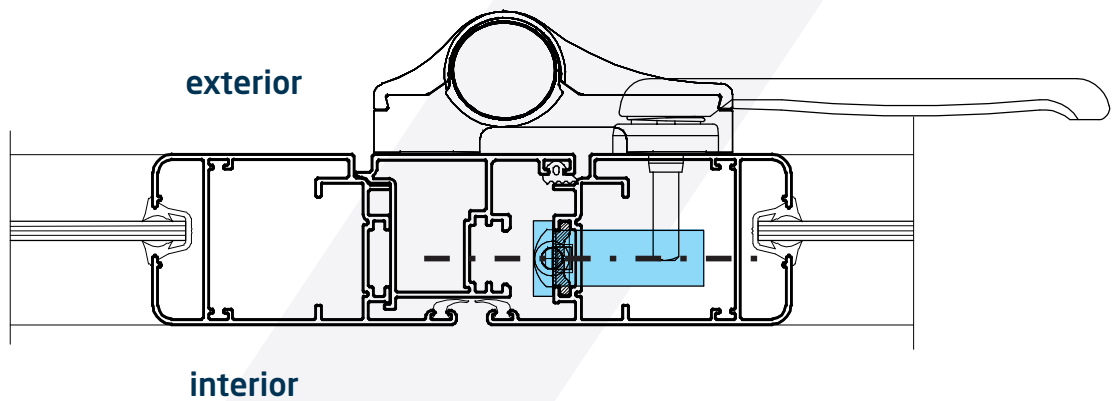
Apertura desde el exterior
