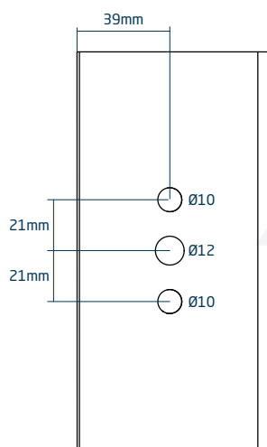
Mecanizado falleba Cód. 2850
