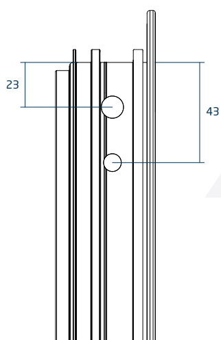
Mecanizado escuadra E-69 Cód. 2850
