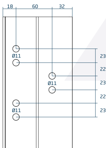
Mecanizado bisagra Loira Cód. 2850 / 2853
