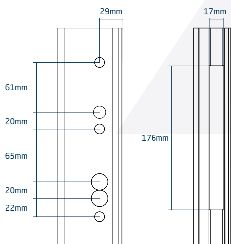
Mecanizado para cerradura con manija recta Cód. 2850
