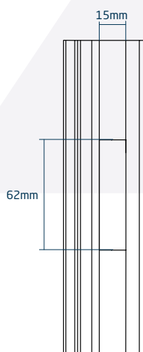
Mecanizado caja bidireccional Cód. 2850
