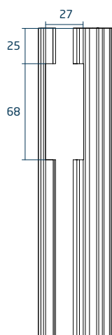
Mecanizado para guía superior Cód. 2872
