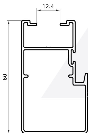
Jamba 0,485 kg/m 02890
