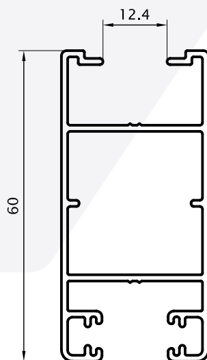
Perfil Refuerzo Umbral 0,138 kg/m 02897
