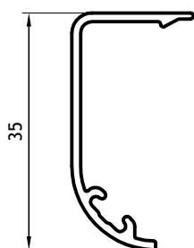
Tapajunta Enclipable 0,250 kg/m 02826 (Barras de 6.05m) 18 Barras por Paquete
