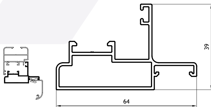
Marco Proyectante Tubular 0,720 kg/m 02824 Barras de 6.05m 8 Barras por Paquete
