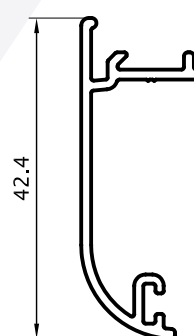
Tapajuntas 0,312 kg/m 09012 Barras de 6.05m 18 Barras por Paquete
