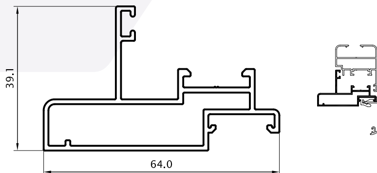
Marco Puerta y Ventana de Abrir Tubular 0,770 kg/m 02825 Barras de 6.05m 8 Barras por Paquete
