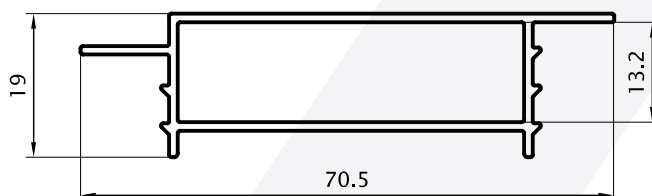
Premarco 0,494 kg/m 00147 Barras de 6.05m 10 Barras por Paquete
