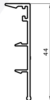
Encuentro Central Interior 0,234 kg/m 02815 Barras de 6.05m
