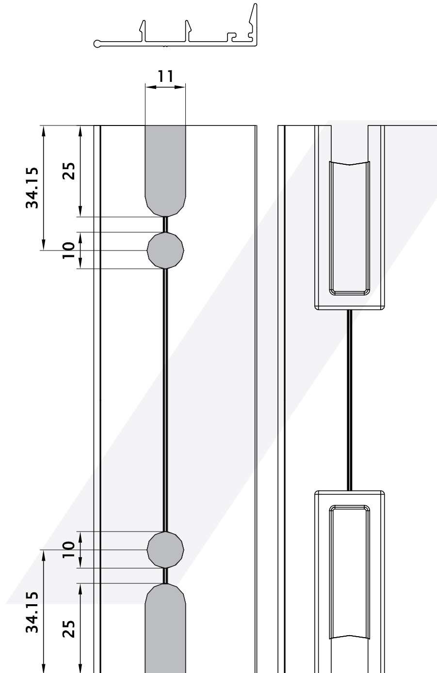
Mecanizados Ranura Larga Encuentro Central Exterior 2815
