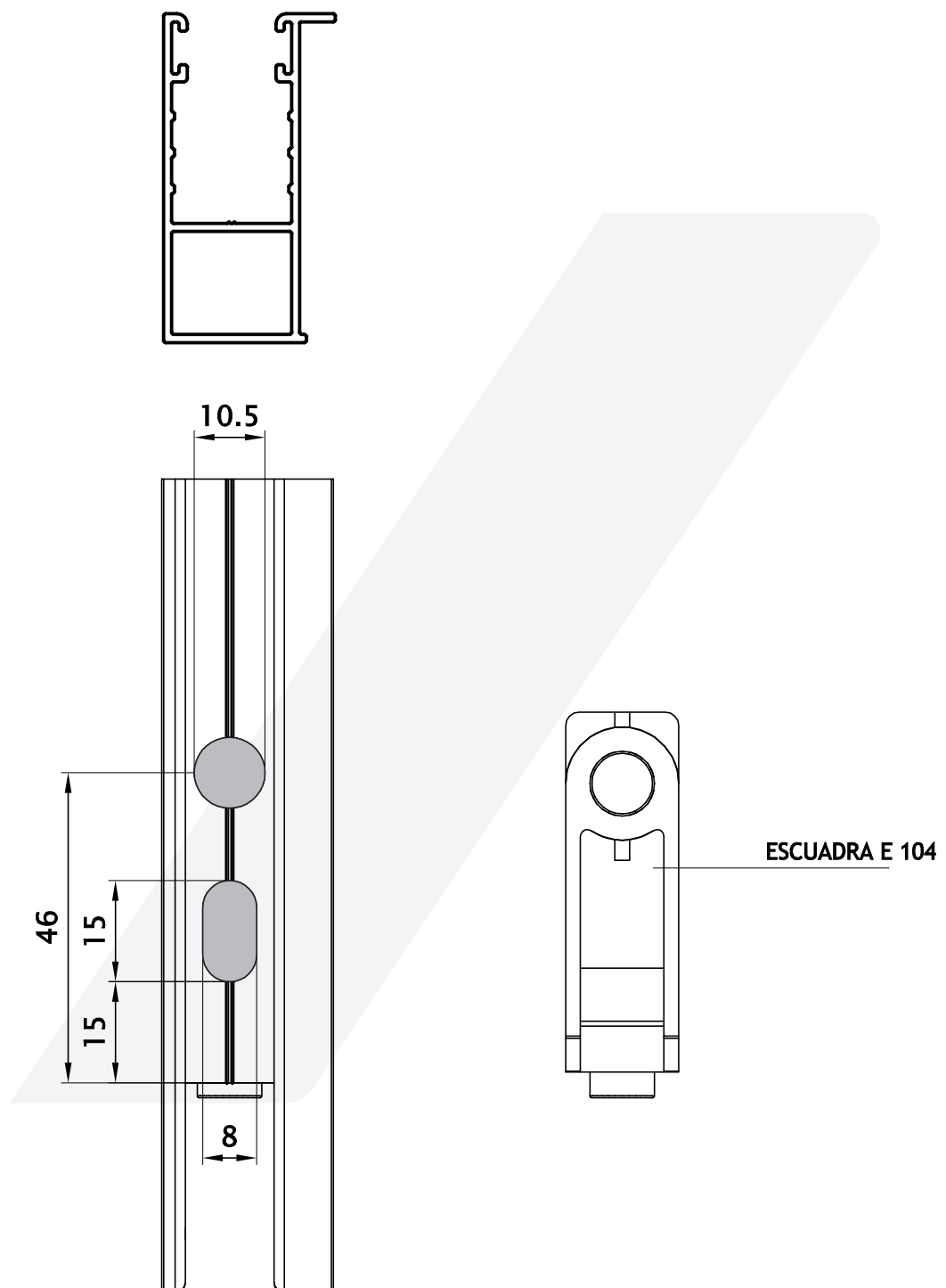
Mecanizado Escuadra E104 Perfil Hoja 2814
