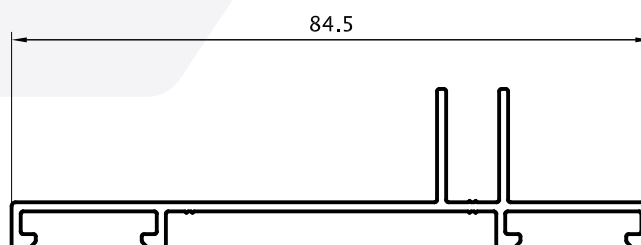
Jamba 0,485 kg/m 02890 Barras de 6.05m
