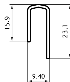
Perfil Refuerzo Umbral 0,145 kg/m 02897 Barras de 6.05m
