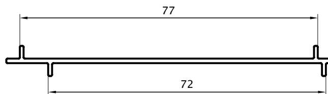
Unión Reducción 180° 0,315 kg/m 02896 Barras de 6.05m
