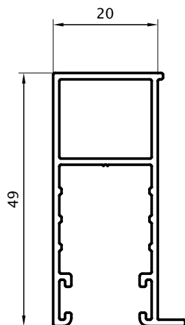
Hoja 50mm 0,514 kg/m 02814 Barras de 6.05m
