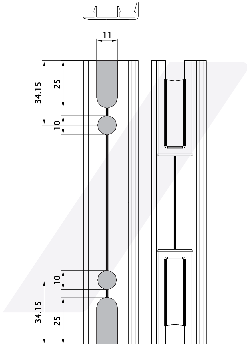
Mecanizados Ranura Larga Encuentro Central Interior 2813
