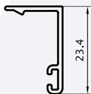
Tapajuntas 0,148 kg/m 02892 Barras de 6.05m 18 Barras por Paquete
