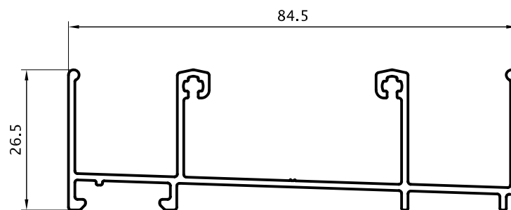
Marco 0,716 kg/m 02891 Barras de 6.05m
