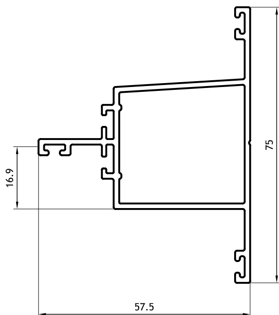
Travesaño 0,922 kg/m 09104 Barras de 6.05m
