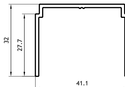
Soporte Columna-Travesaño 0,418 kg/m 09109 Barras de 6.05m
