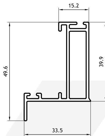
Hoja con Ala 0,564 kg/m 09107 Barras de 6.05m
