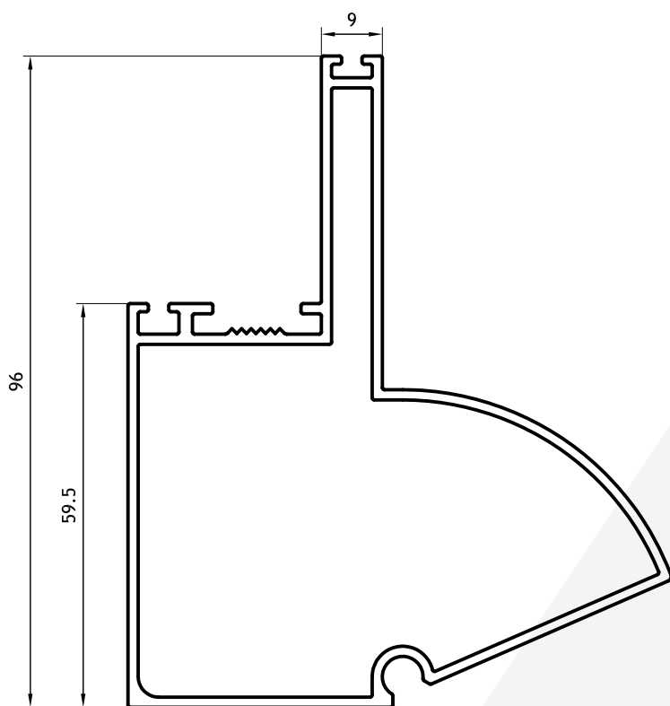
1/2 Columna Rotador Hembra 96mm 1,440 kg/m 09102 Barras de 6.20m
