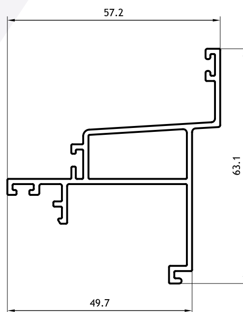
Travesaño Inferior 0,775 kg/m 09116 Barras de 6.05m
