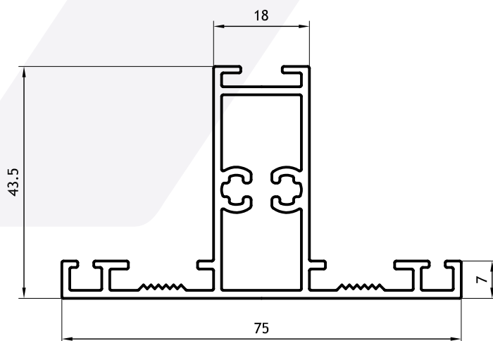
Columna 43mm - Travesaño 1,040 kg/m 09118 Barras de 6.05m
