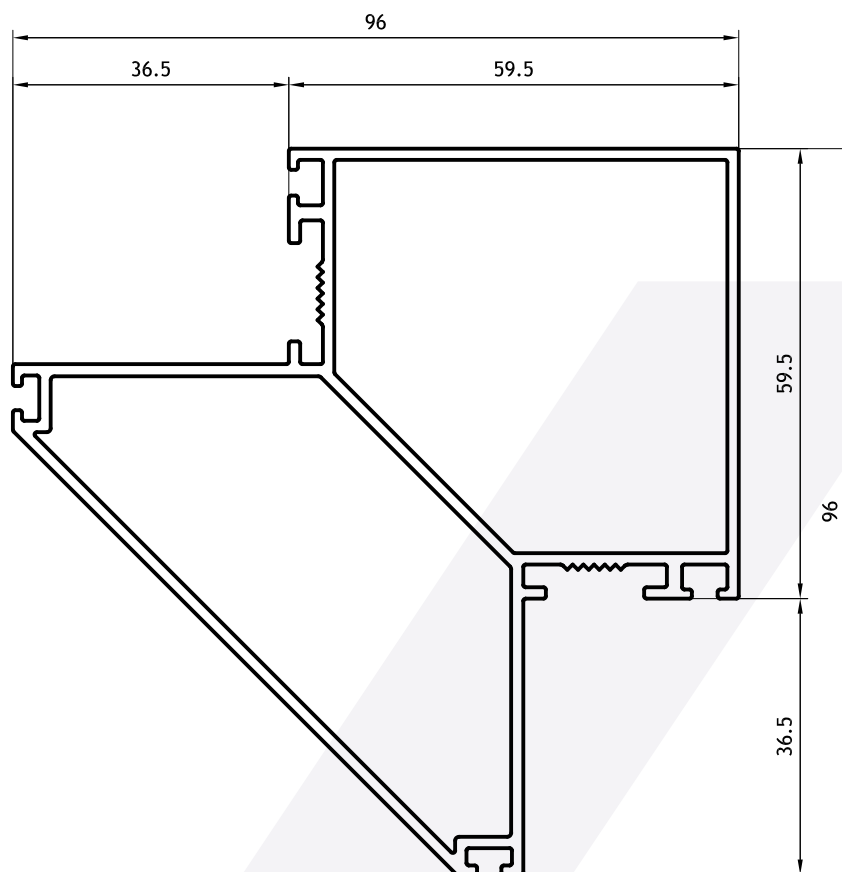
Columna Esquina 96mm 1,830 kg/m 09114 Barras de 6.05m
