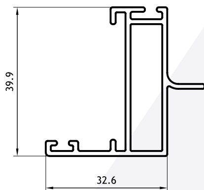
Hoja DVH 0,562 kg/m 09108 Barras de 6.05m
