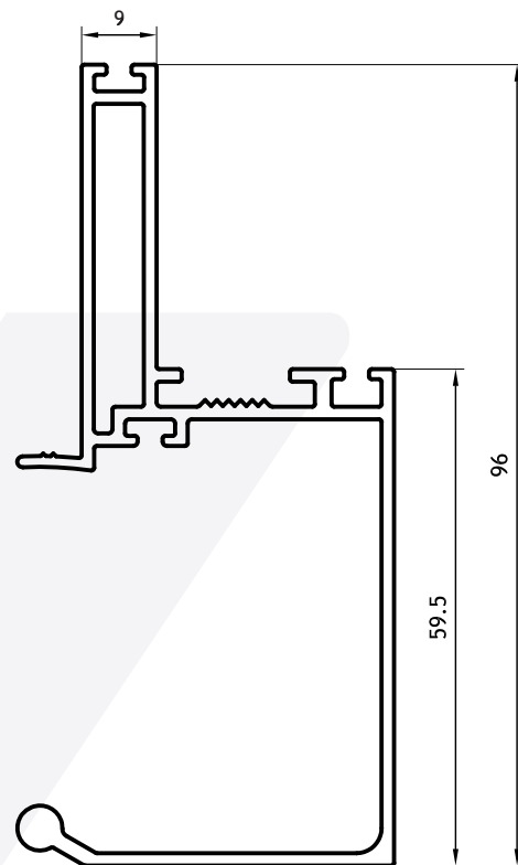
1/2 Columna Rotador Macho 96mm 1,154 kg/m 09103 Barras de 6.20m
