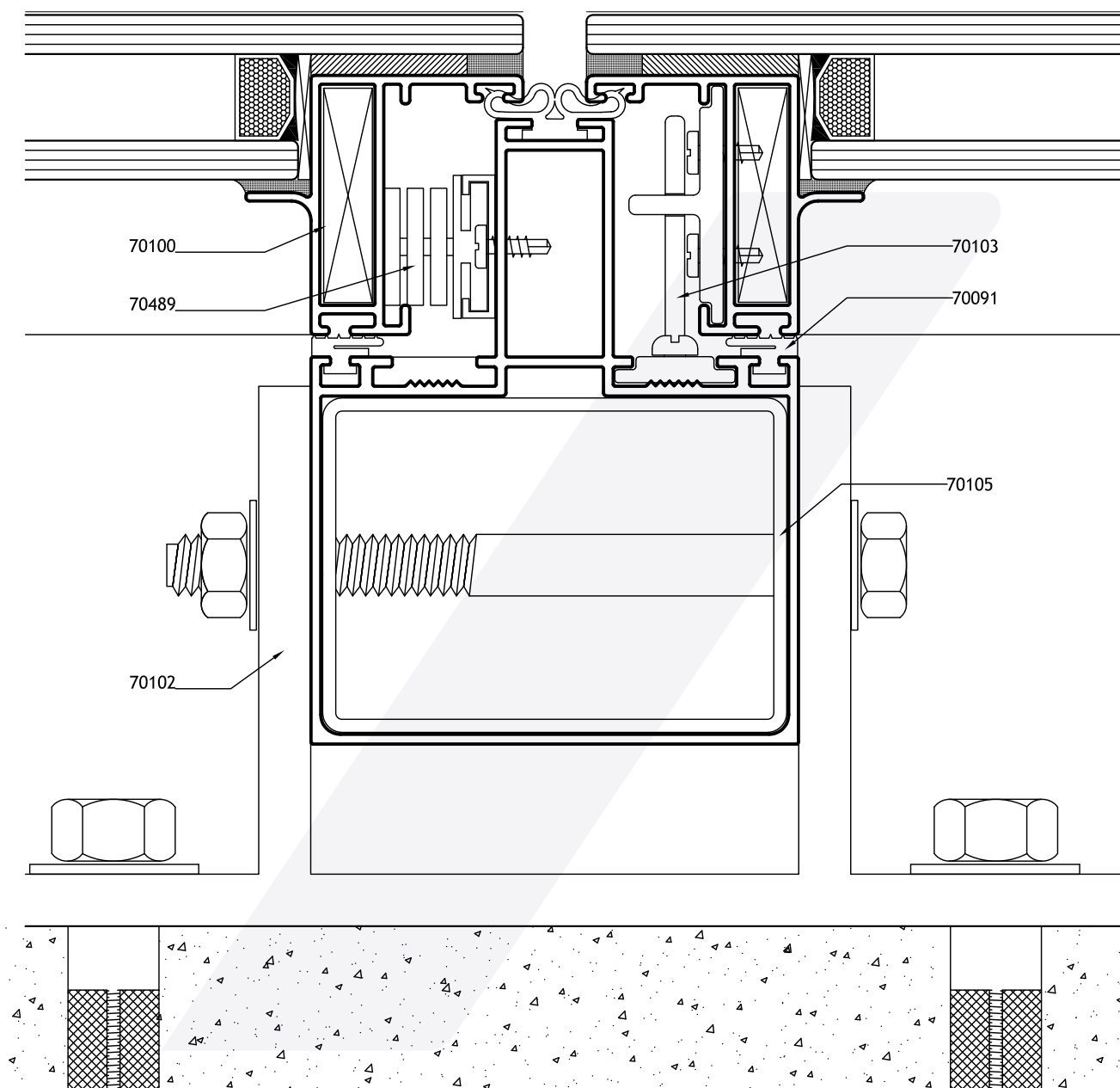
Corte Horizontal Detalle Columna 96mm con Hoja Proyectante y Paño Fijo
