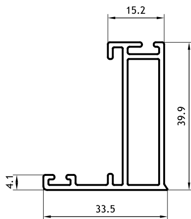
Hoja 0,527 kg/m 09106 Barras de 6.05m
