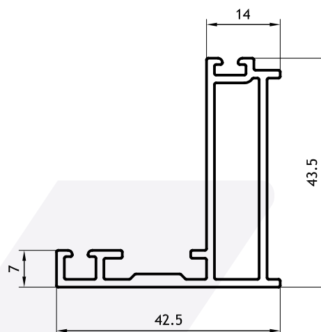
Travesaño Superior-Inferior 0,687 kg/m 09105 Barras de 6.05m
