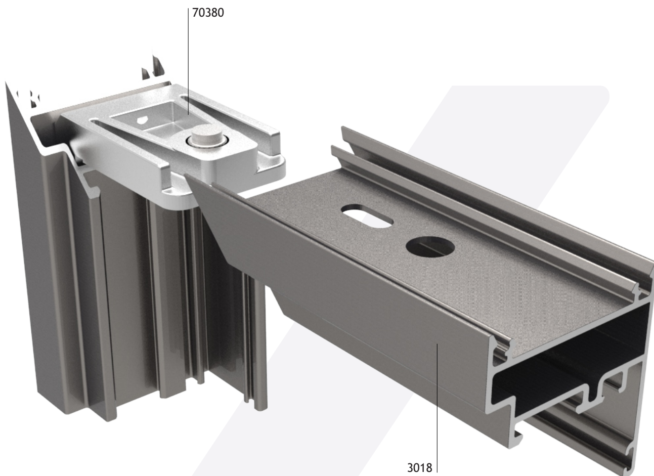
DETALLE MECANIZADO MARCO 3018 - ALOJAMIENTOS PARA ESCUADRA 70380
