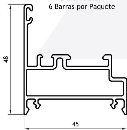
Marco 0,725 kg/m 03018 Barras de 6.05m 6 Barras por Paquete
