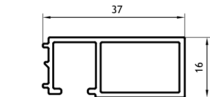
Premarco 37mm 0,371 Kg/m 03015 Barras de 6.20m 10 Barras por Paquete
