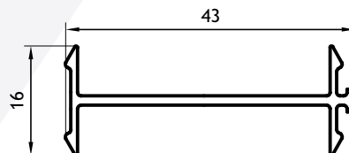
Unión Marco 180° 0,262 Kg/m 03017 Barras de 6.05m 20 Barras por Paquete
