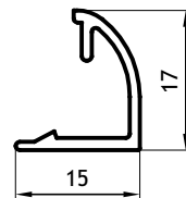
Contravidrio Curvo DVH 0,134 Kg/m 03213 Barras de 6.05m 20 Barras por Paquete
