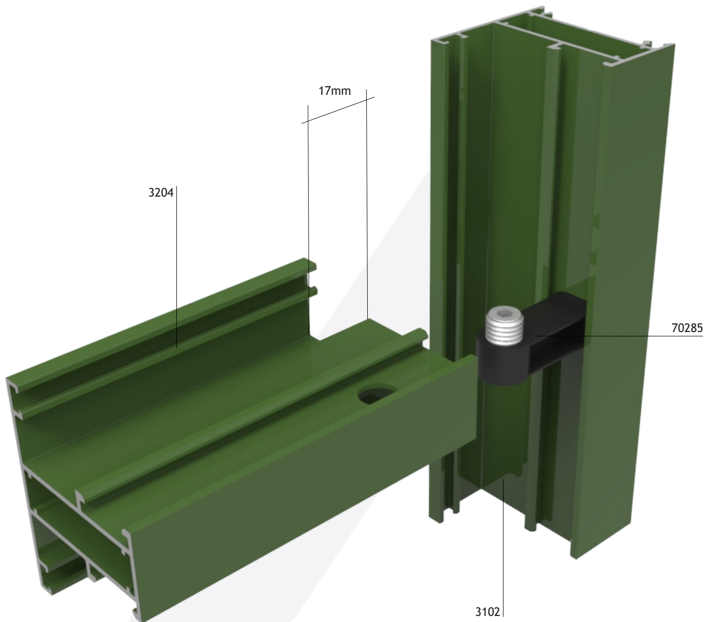
DETALLE MECANIZADO TRAVESAÑO 3204 ENCUENTRO Y MARCO 3102 CON SOPORTE ANGOSTO E-71
