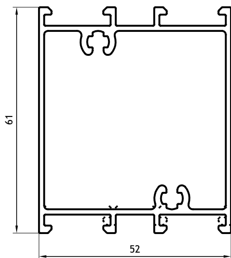
Travesaño Hoja 1,134 Kg/m 03100 Barras de 6.05m 4 Barras por Paquete
