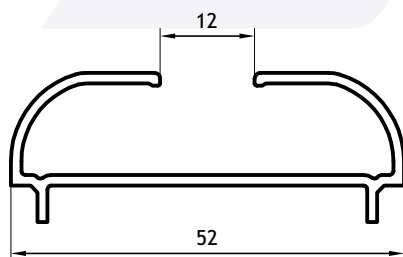
Contravidrio 0,447 Kg/m 03103 Barras de 6.05m 10 Barras por Paquete
