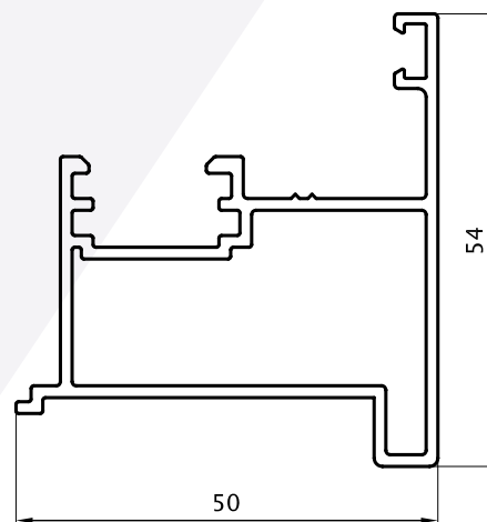
Encuentro Central 0,827 Kg/m 03105 Barras de 6.05m 6 Barras por Paquete
