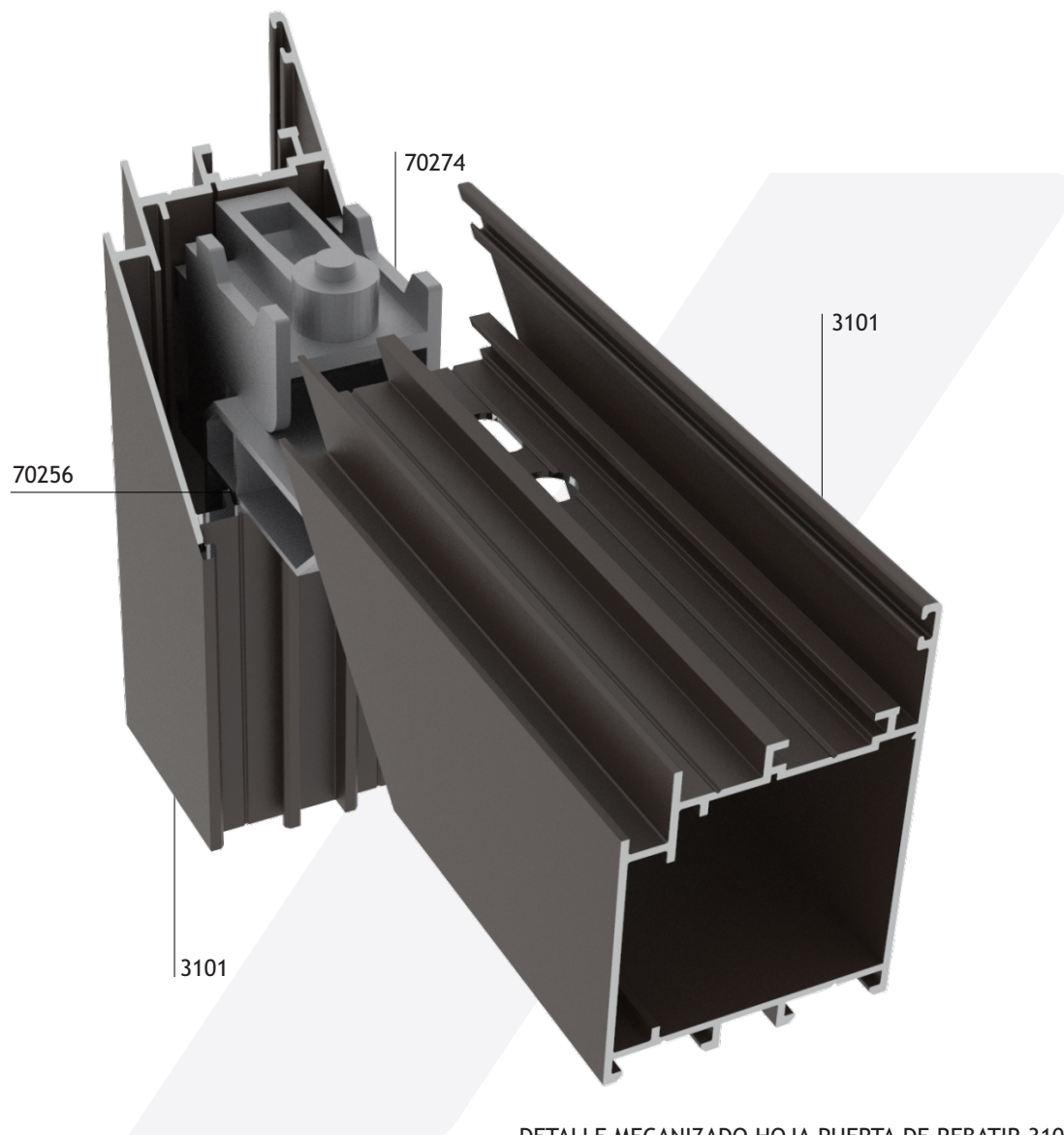
DETALLE MECANIZADO HOJA PUERTA DE REBATIR 3101 ALOJAMIENTO ESCUADRA 70274 + ESCUADRA SUPLEMENTARIA 70256
