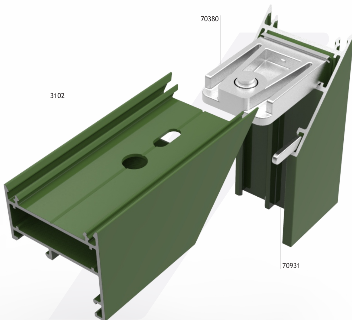
DETALLE MECANIZADO MARCO 3102 - ALOJAMIENTOS PARA ESCUADRA 70380
