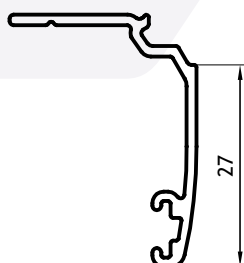
TapaJunta Curvo 0,375 Kg/m 03024 Barras de 6.05m 10 Barras por Paquete
