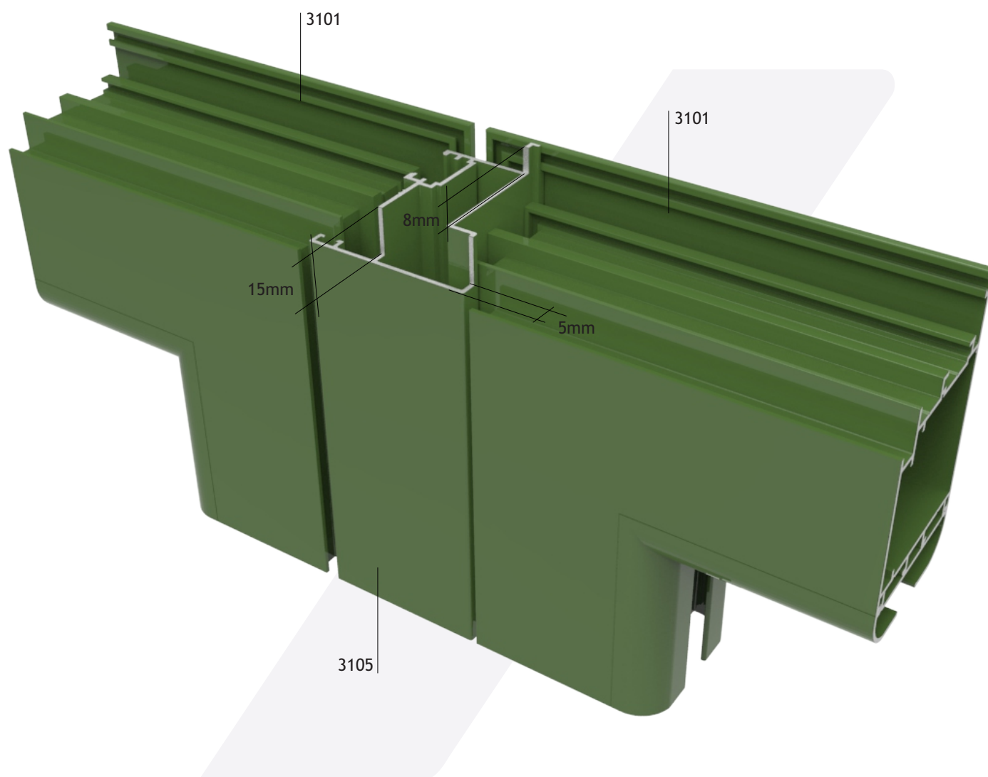
DETALLE MECANIZADO ENCUENTRO CENTRAL 3105 (nota importante: las medidas expresadas son estimativas y pueden variar en relación a la marca de los accesorios utilizados)
