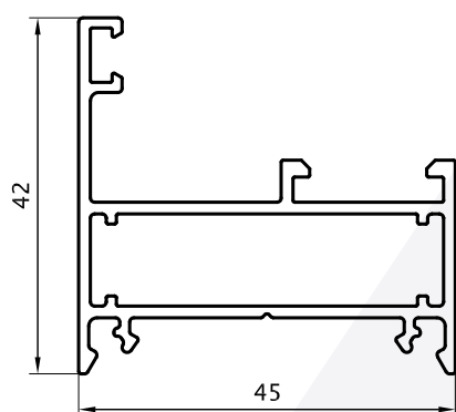
Marco Puerta 0,710 Kg/m 03102 Barras de 6.20m 6 Barras por Paquete
