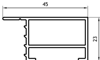
Premarco 0,460 Kg/m 03022 Barras de 6.05m 10 Barras por Paquete
