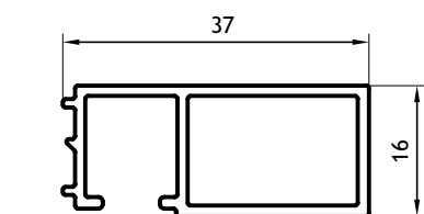
Premarco 37mm 0,371 Kg/m 03015 Barras de 6.20m 10 Barras por Paquete
