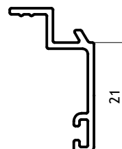
TapaJunta 0,180 Kg/m 02810 Barras de 6.05m 20 Barras por Paquete
