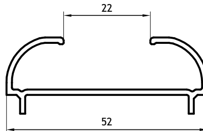
Contravidrio DVH 0,409 Kg/m 03104 Barras de 6.05m 10 Barras por Paquete
