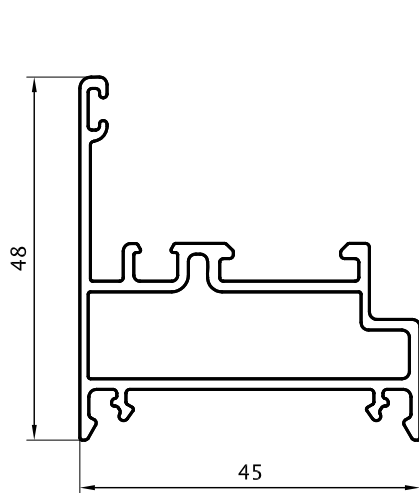
Marco 0,725 kg/m 03018 (Barras de 6.05m)
