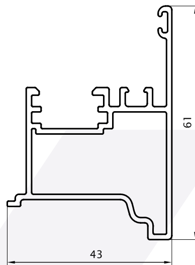
Encuentro Central 0,829 kg/m 03020 (Barras de 6.05m)
