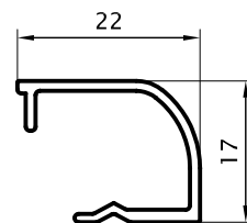
Contravidrio Curvo 0,180 Kg/m 03212 (Barras de 6.05m)
