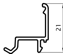
Contravidrio 30mm 0,160 Kg/m 03214 (Barras de 6.05m)
