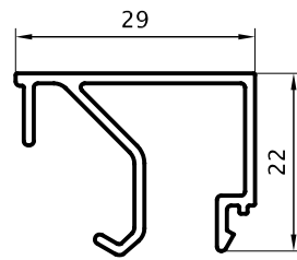
Contravidrio Recto 0,298 Kg/m 03210 (Barras de 6.05m)
