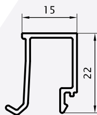
Contravidrio Recto DVH 0,214 Kg/m 03211 (Barras de 6.05m)
