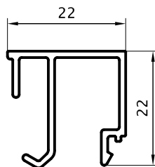
Contravidrio Recto Alojamiento 17mm 0,258 Kg/m 03209 (Barras de 6.05m)
