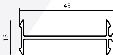
Unión Marco 180° 0,262 Kg/m 03017 (Barras de 6.05m)
