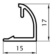
Contravidrio Curvo DVH 0,134 Kg/m 03213 (Barras de 6.05m)
