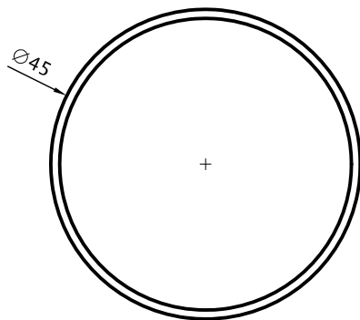
Caño Redondo para Rotador de Grados 0,490 Kg/m 01332 (Barras de 6.05m)
