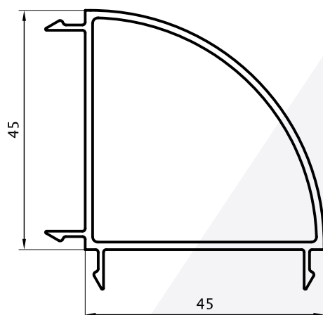
Unión Marco 90° 0,694 Kg/m 03016 (Barras de 6.05m)
