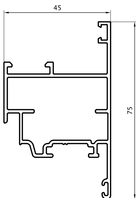
Hoja Ventiluz 0,950 Kg/m 03038 (Barras de 6.05m)
