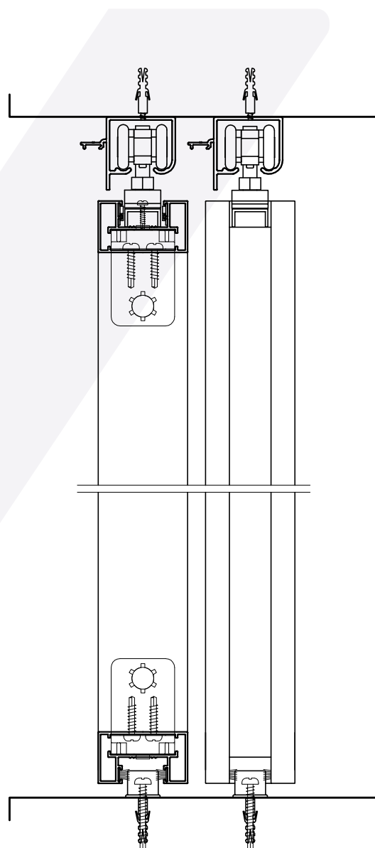
SECCIÓN VERTICAL 1-1 escala 1:3
