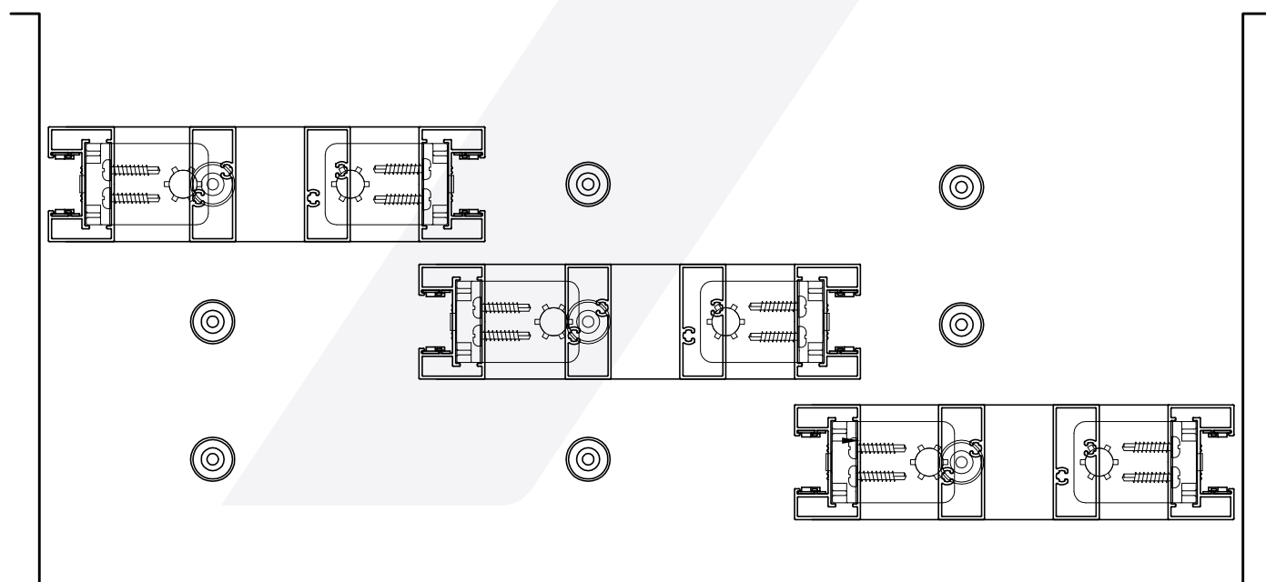
SECCIÓN HORIZONTAL 2-2
