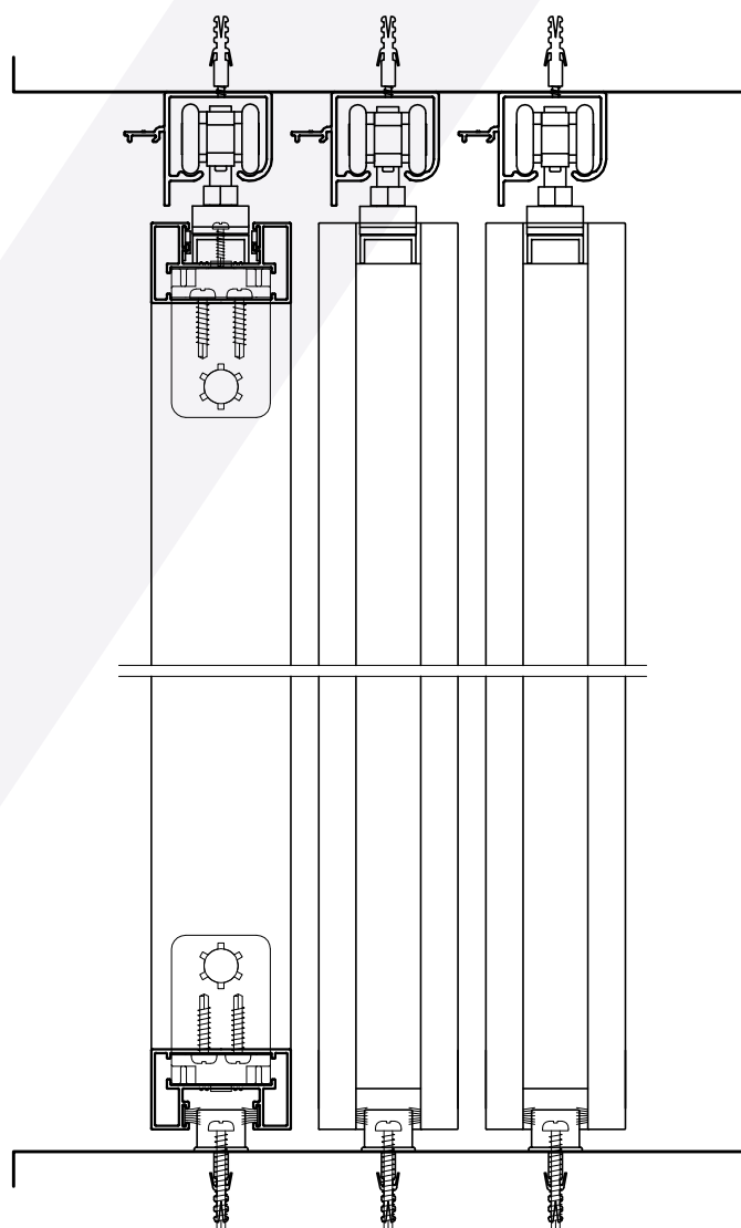
SECCIÓN VERTICAL 1-1
