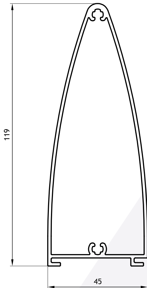
Puntera Parasol Tubular 1,332 Kg/m 09400 Barras de 6.20m
