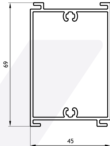
Núcleo Central Parasol Tubular 1,102 Kg/m 09401 Barras de 6.20m
