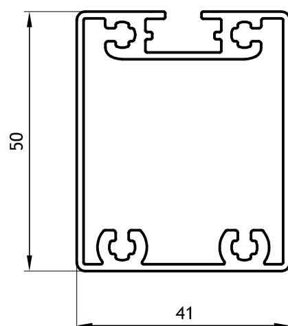
Columna 1,090 Kg/m 09203 Barras de 6.05m
