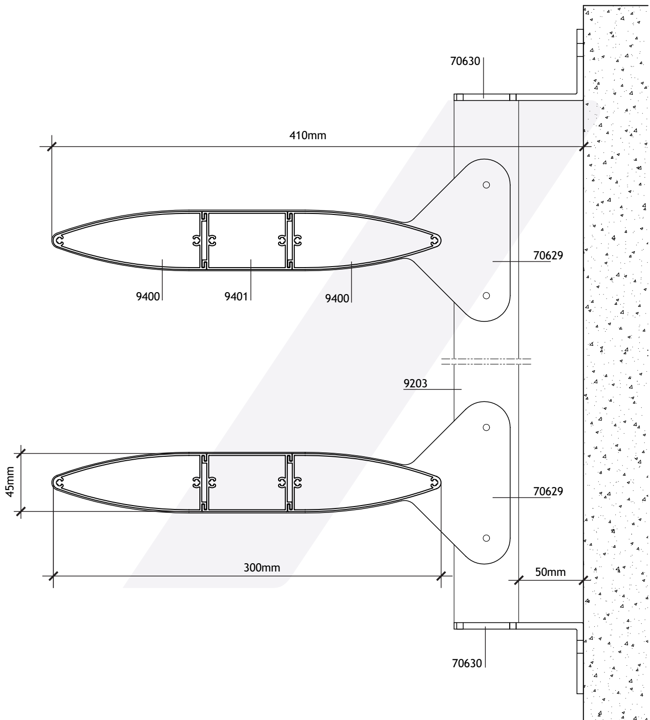
SECCIÓN VERTICAL
