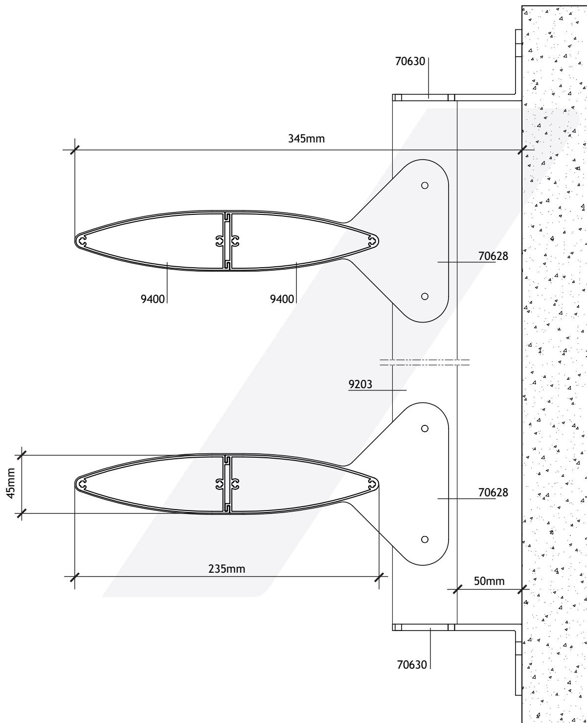
SECCIÓN VERTICAL
