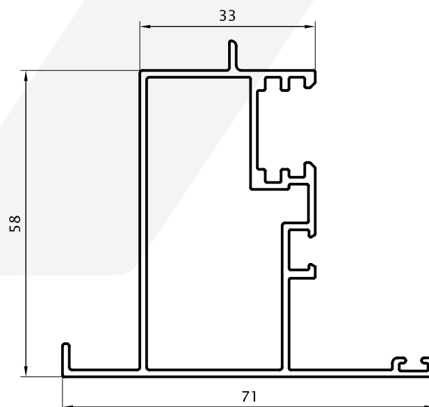
Encuentro Central 1,020 Kg/m 08105 Barras de 6.05m
