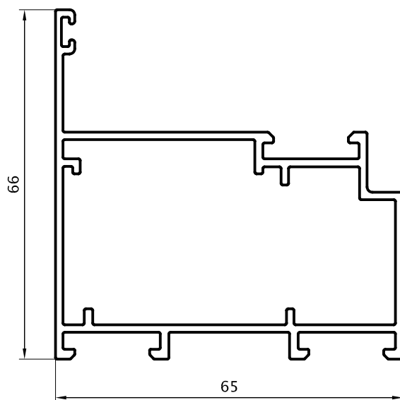
Marco Puerta de Abrir 1,095 Kg/m 08102 Barras de 6.05m
