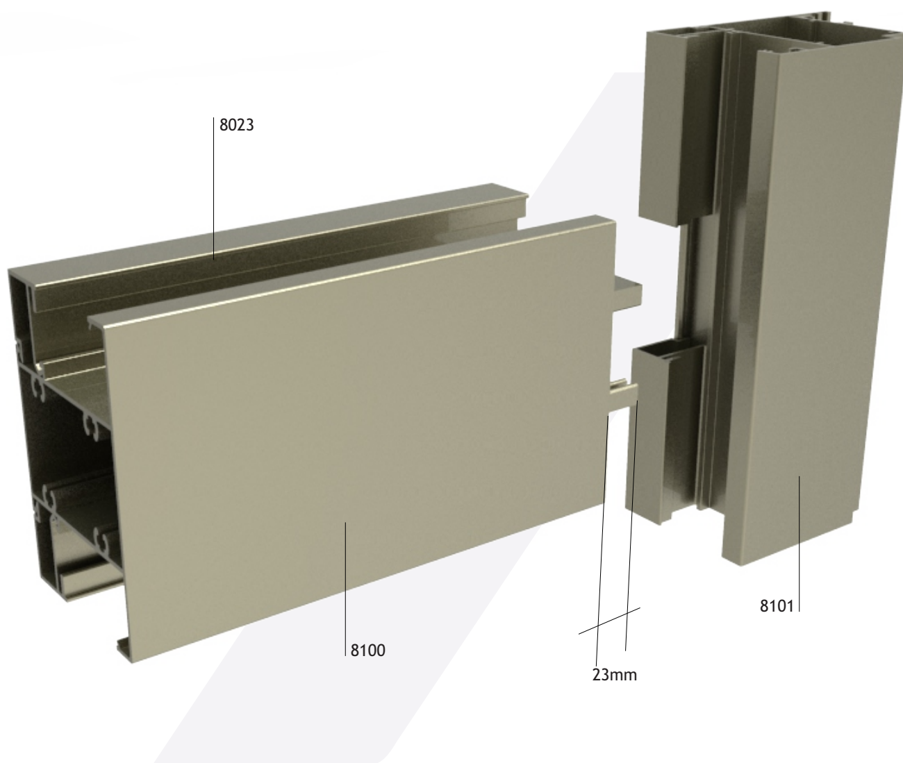
Detalle mecanizados Travesaño 8100
