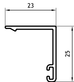
Tapajunta 25mm 0,198 Kg/m 08012 Barras de 6.05m
