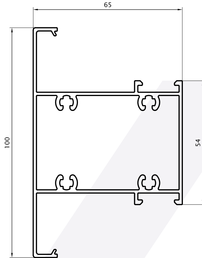
Travesaño Puerta de Abrir 1,550 Kg/m 08100 Barras de 6.05m
