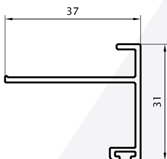
Zócalo Puerta de Abrir 0,310 Kg/m 08104 Barras de 6.05m
