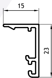
Tapajunta 23mm 0,185 Kg/m 08013 Barras de 6.05m
