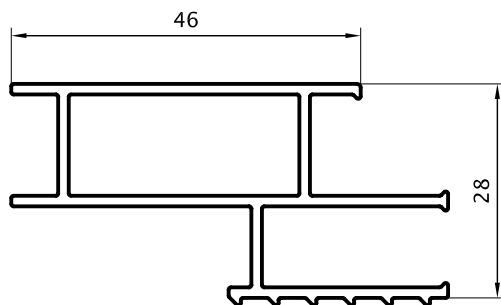
Premarco Pasacable 65mm 0,740 Kg/m 08029 Barras de 6.05m
