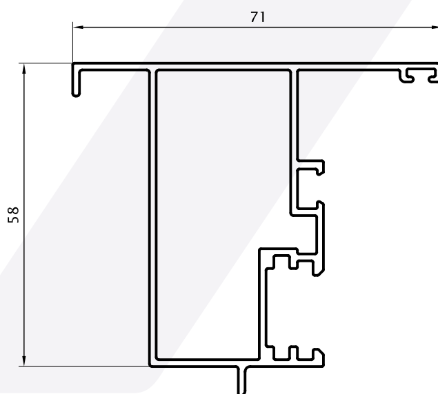
Encuentro Central 0,985 Kg/m 08105 Barras de 6.05m
