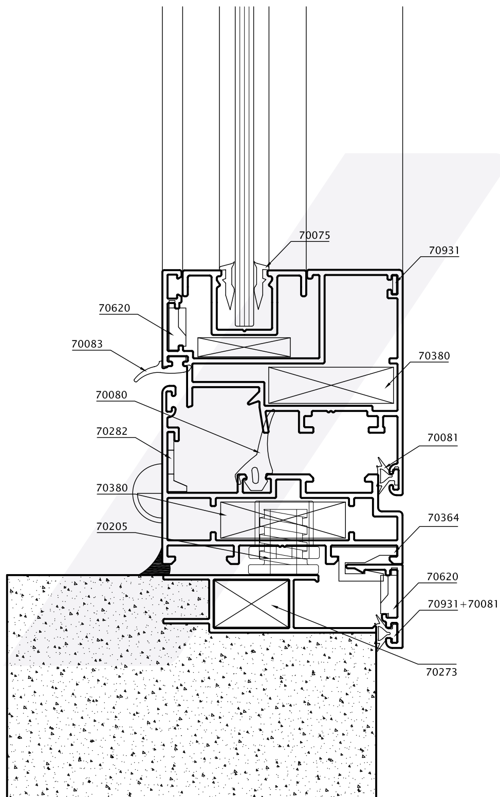
Detalle encuentro inferior
