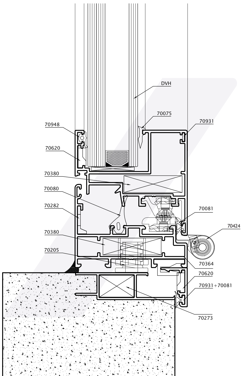
Detalle encuentro lateral bisagra Escala 1:1
