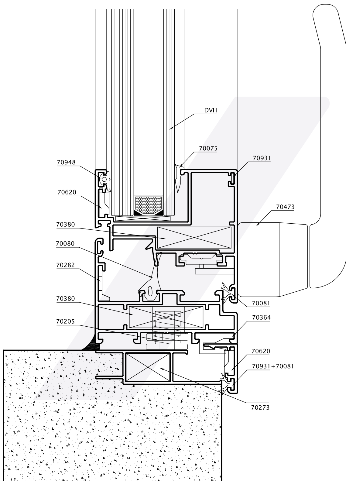
Detalle encuentro lateral falleba
