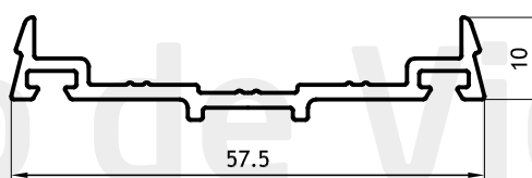
Contratapa 0,408 kg/m 09501 Barras de 6.05m
