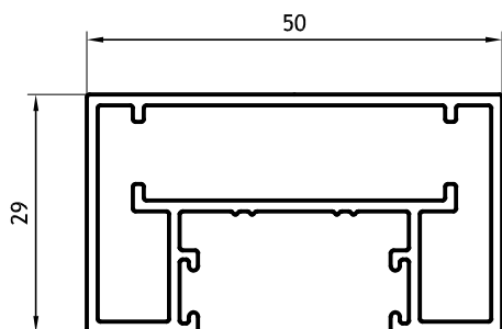
Hoja Celosía Corrediza 0,753 Kg/m 03220 Barras de 6.05m
