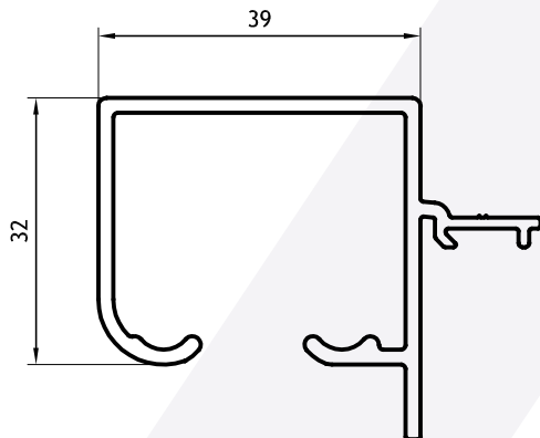
Guía Superior 0,730 Kg/m 02872 Barras de 6.05m
