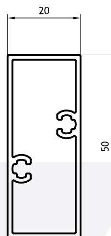
Lama Celosía Corrediza 0,577 Kg/m 03221 Barras de 6.05m
