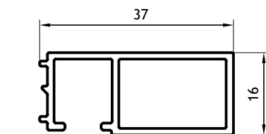
(S) Premarco 37mm 0,371 Kg/m 03015 Barras de 6.20m 10 Barras por Paquete
