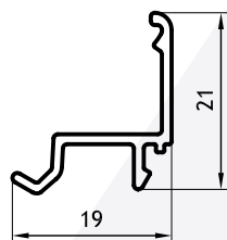
Contravidrio 30mm 0,160 Kg/m 03214 Barras de 6.05m
