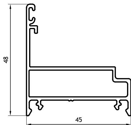
Marco Ventana Desplazable 0,650 Kg/m 03099 Barras de 6.05m 6 Barras por Paquete
