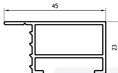
(S) Premarco 0,460 Kg/m 03022 Barras de 6.05m 10 Barras por Paquete
