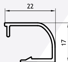
S Contravidrio Curvo 0,180 Kg/m 03212 Barras de 6.05m 20 Barras por Paquete
