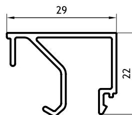
S Contravidrio Recto 0,298 Kg/m 03210 Barras de 6.05m 20 Barras por Paquete
