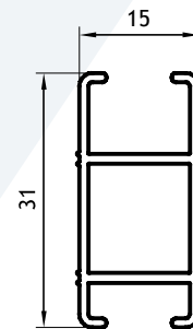
Hoja 0,290 Kg/m 00554 Barras de 6.05m 12 Barras por Paquete
