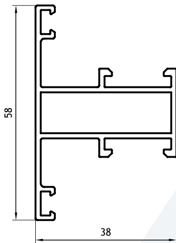
Travesaño Curvo 0,726 Kg/m 03203 Barras de 6.05m 6 Barras por Paquete
