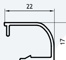
Contravidrio Recto 0,298 Kg/m 03210 Barras de 6.05m 20 Barras por Paquete
