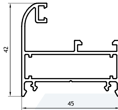
Marco Curvo 0,748 Kg/m 03201 Barras de 6.05m 6 Barras por Paquete
