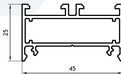
Marco Doble Contravidrio 0,652 Kg/m 03202 Barras de 6.05m 6 Barras por Paquete
