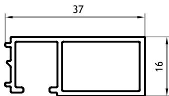
Premarco 37mm 0,371 Kg/m 03015 Barras de 6.20m 10 Barras por Paquete
