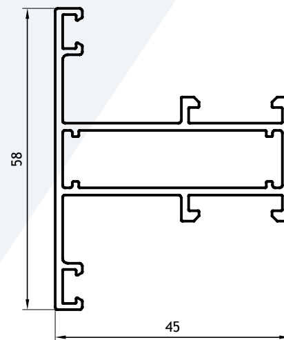
Travesaño Recto 0,797 Kg/m 03204 Barras de 6.05m 6 Barras por Paquete
