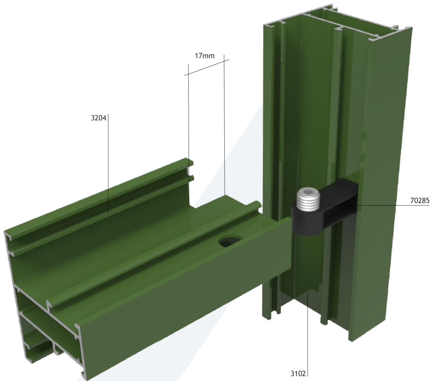
DETALLE MECANIZADO TRAVESAÑO 3204 ENCUESTRO Y MARCO 3102 CON SOPORTE ANGOSTO E-71
