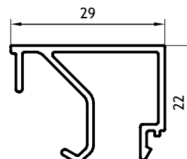
Contravidrio Recto 0,298 Kg/m 03210 Barras de 6.05m 20 Barras por Paquete
