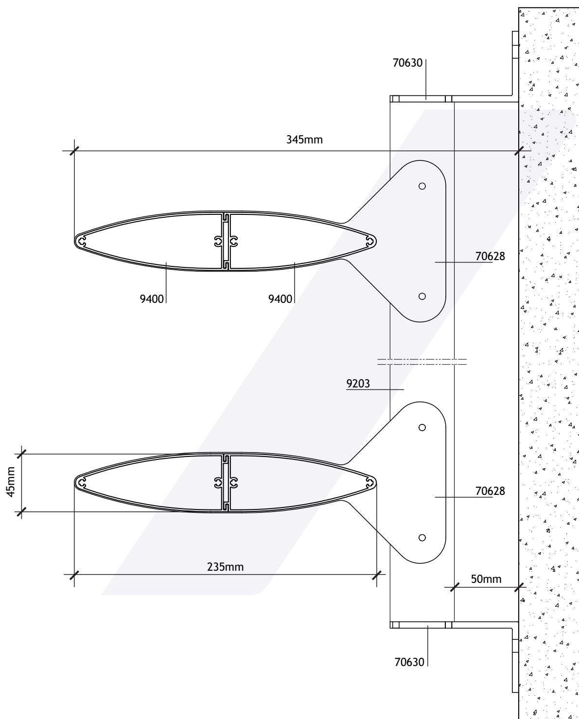
SECCIÓN VERTICAL
