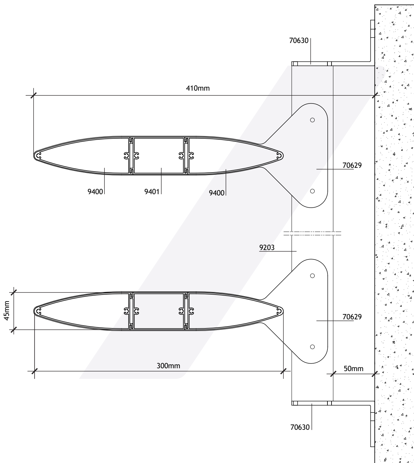
SECCIÓN VERTICAL
