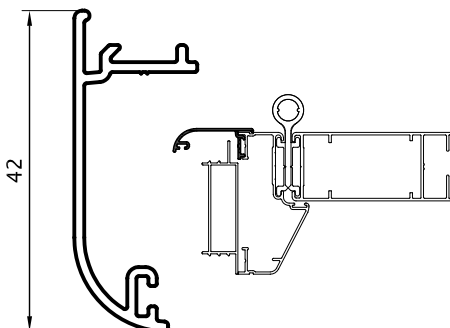
Tapajuntas 0,312 Kg/m 09012 (Barras de 6.05m) 18 Barras por Paquete
