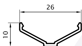
Moldura Vidrio Repartido 0,112 Kg/m 00267 (Barras de 6.05m) 10 Barras por Paquete
