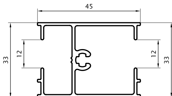
Travesaño Puerta F 45mm 0,635 kg/m 00180 (Barras de 6.05m) 9 Barras por Paquete
