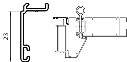
Tapajuntas 0,148 Kg/m 09013 (Barras de 6.05m) 18 Barras por Paquete
