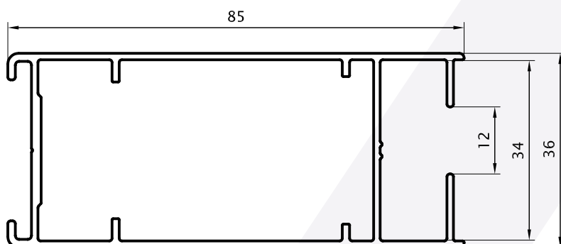
Parante Puerta F 85mm 1,064 kg/m 00178 (Barras de 6.20m) 4 Barras por Paquete
