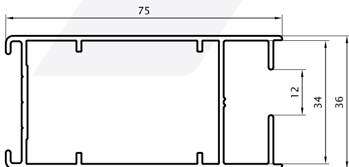
Parante Puerta F 75mm 0,957 kg/m 00179 (Barras de 6.20m) 4 Barras por Paquete
