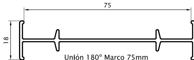
Unión 180° Marco 75mm 0,459 Kg/m 00106 (Barras de 6.05m)
