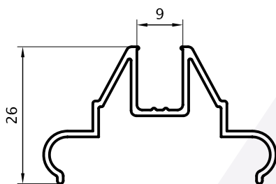
Vidrio Repartido Puerta F 0,330 Kg/m 00256 (Barras de 6.05m) 12 Barras por Paquete
