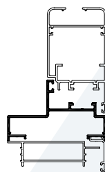
Marco Puerta y Ventana de Abrir 0,720 kg/m 02851 Barras de 6.05m 8 Barras por Paquete
