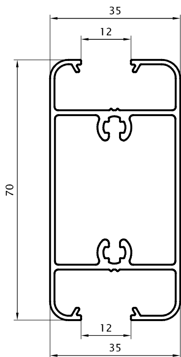
Travesaño 70 mm 1,020 kg/m 02881 Barras de 6.05m 18 Barras por Paquete
