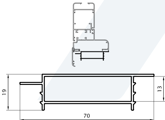
Premarco 0,494 kg/m 00147 Barras de 6.05m 10 Barras por Paquete
