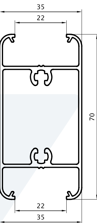
Travesaño 70 mm DVH 0,961 kg/m 02882 Barras de 6.05m 18 Barras por Paquete
