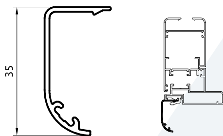
Tapajunta Enclipable 0,250 kg/m 02826 (Barras de 6.05m) 18 Barras por Paquete
