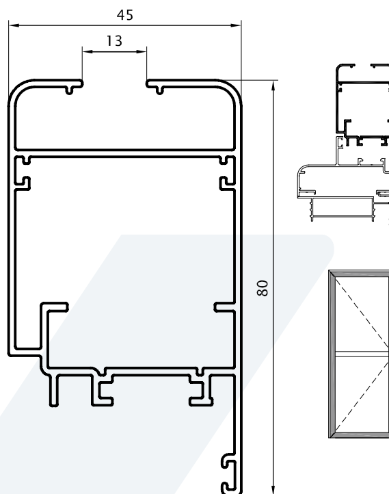
Hoja Puerta de Abrir 1,099 kg/m 02850 Barras de 6.05m 4 Barras por Paquete
