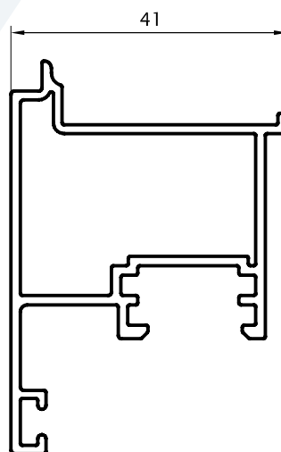
Encuentro Hojas de Abrir 0,754 kg/m 02853 Barras de 6.05m 6 Barras por Paquete
