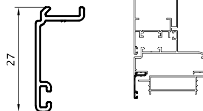
Tapajuntas 0,148 kg/m 09013 Barras de 6.05m 18 Barras por Paquete
