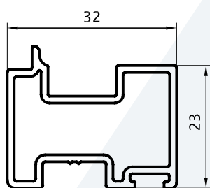
Zócalo Puerta de Abrir 0,375 kg/m 02852 Barras de 6.05m 10 Barras por Paquete
