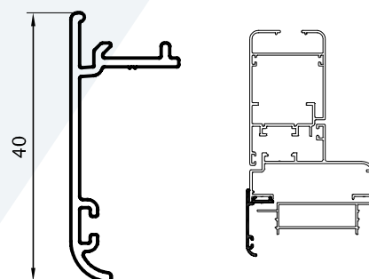
Tapajuntas 0,251 kg/m 09011 Barras de 6.05m 18 Barras por Paquete
