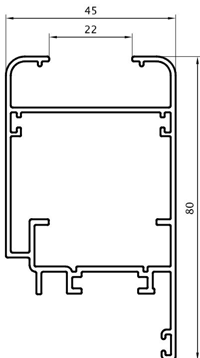
Hoja Puerta de Abrir DVH 1,080 kg/m 02830 Barras de 6.05m 4 Barras por Paquete
