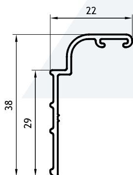
Doble Contacto 0,214 kg/m 00205 (Barras de 6.05m) 20 Barras por Paquete
