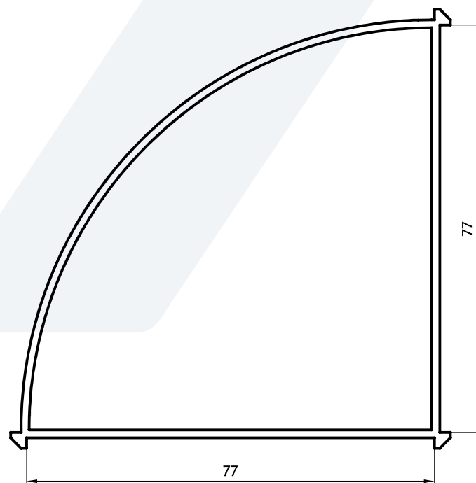
Unión 90° Marco 75mm 1,205 Kg/m 00330 (Barras de 6.05m)
