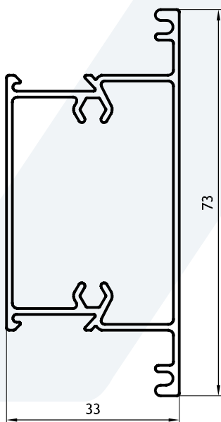
Travesaño 72.5mm 0,740 kg/m 00203 (Barras de 6.05m) 4 Barras por Paquete
