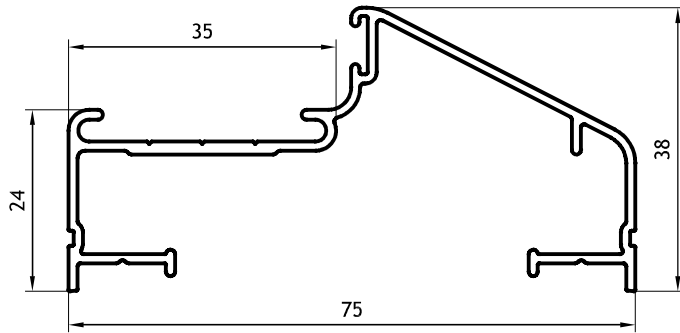
Marco 0,629 kg/m 00200 (Barras de 6.20m) 8 Barras por Paquete
