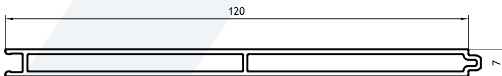
Tablilla Tubular Liso 120mm (8 tablillas x metro lineal) 0,867 Kg/m 00093 (Barras de 6.05m) 4 Barras por Paquete
