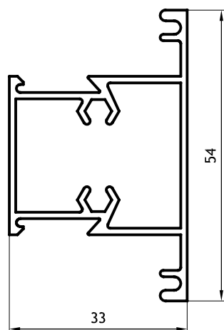
Travesaño 54mm 0,679 kg/m 00202 (Barras de 6.05m) 6 Barras por Paquete
