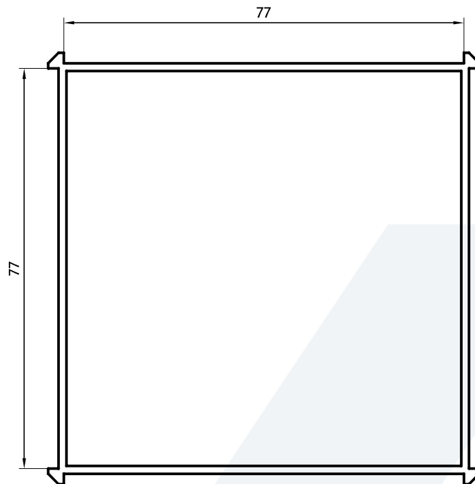
Unión Cuadrangular Marco 75mm 1,360 Kg/m 00094 (Barras de 6.05m)
