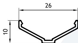
Moldura Vidrio Repartido 0,112 Kg/m 00267 (Barras de 6.05m) 10 Barras por Paquete
