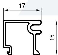
Contravidrio 0,163 kg/m 00108 (Barras de 6.05m) 30 Barras por Paquete
