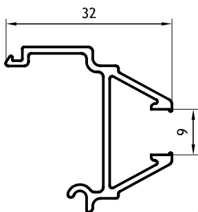
Vidrio Repartido Perimetral Contravidrio 0,322 Kg/m 00250 (Barras de 6.05m) 12 Barras por paquete
