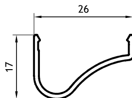
Moldura Curva 0,168 Kg/m 00266 (Barras de 6.05m) 10 Barras por Paquete
