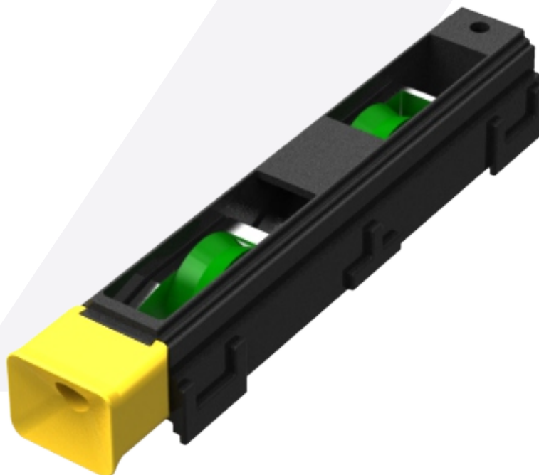
70712 Rodamiento Giesse Regulable Carrera 2 p/perfil 3014-3023 x 4 unidades
