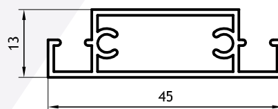
Travesaño 0,422 kg/m 00115 Barras de 6.05m 10 Barras por Paquete
