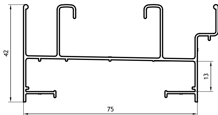
Marco 0,760 kg/m 00101 Barras de 6.05m 6 Barras por Paquete
