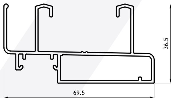
Marco Corredizo Tubular 0,880 kg/m 02823 (Barras de 6.05m) 6 Barras por Paquete
