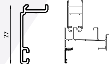
Tapajuntas 0,148 kg/m 09013 Barras de 6.05m 18 Barras por Paquete
