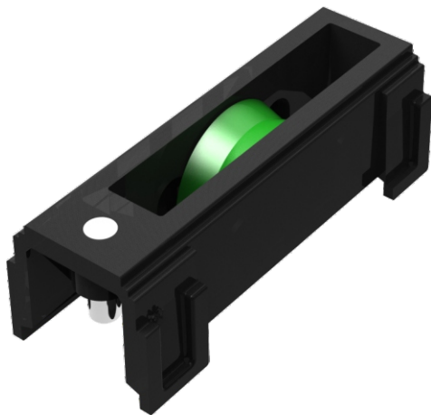
70711 Rodamiento Giesse Rueda Fija Carrera p/perfil 3014-3023 x 4 unidades
