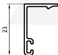
Tapajuntas 0,148 kg/m 02892 Barras de 6.05m
