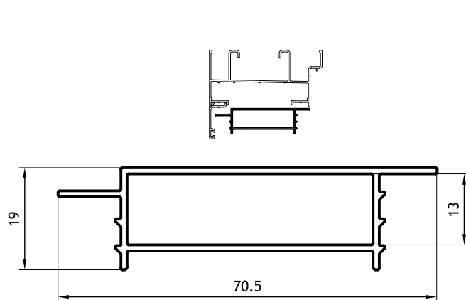
Premarco 0,494 kg/m 00147 Barras de 6.05m 10 Barras por Paquete
