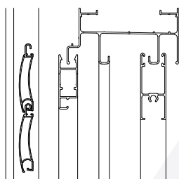
Tablilla Cortina de Enrollar 0,426 kg/m 00413 Barras de 6,05m 10 Barras por Paquete
