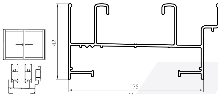
Marco 0,920 kg/m 09001 Barras de 6,05m 6 Barras por Paquete
