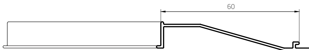
Tablilla Postigón 60mm (15 tablillas / metro lineal) 0,248 kg/m 00420 Barras de 6,05m 15 Barras por Paquete
