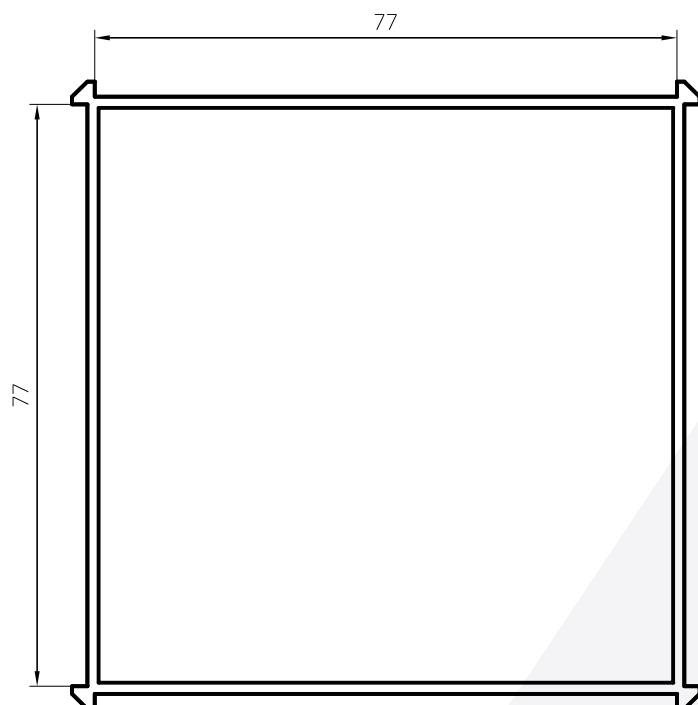
Unión Cuadrangular Marco 75mm 1,360 kg/m 00094 Barras de 6,05m 2 Barras por Paquete
