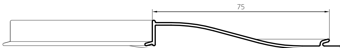
Tablilla Postigón 75mm (13 tablillas / metro lineal) 0,301 kg/m 00417 Barras de 6,05m 15 Barras por Paquete
