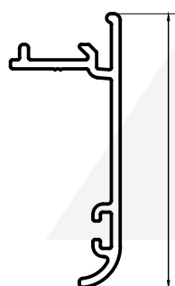
Tapajuntas Recto 0,251 kg/m 09011 Barras de 6,05m 18 Barras por Paquete
