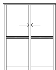
Parante Lateral Curves 0,524 kg/m 00173 Barras de 6,05m 8 Barras por Paquete
