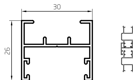
Cierre Central 4 Hojas en 2 Guías 0,320kg/m 00119 Barras de 6,05m 12 Barras por Paquete
