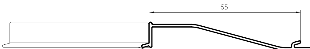
Tablilla Postigón 65mm (15 tablillas / metro lineal) 0,265 kg/m 00418 Barras de 6,05m 15 Barras por Paquete
