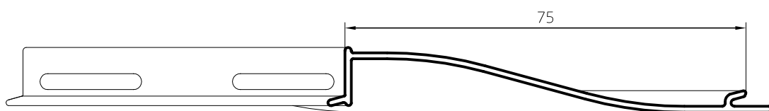
Tablilla Postigón 75mm troquelada (13 tablillas / metro lineal) 0,301 kg/m 00427 Barras de 6,05m 15 Barras por Paquete
