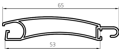
Tablilla Cortina de Enrollar 0,426 kg/m 00413 Barras de 6,05m 10 Barras por Paquete
