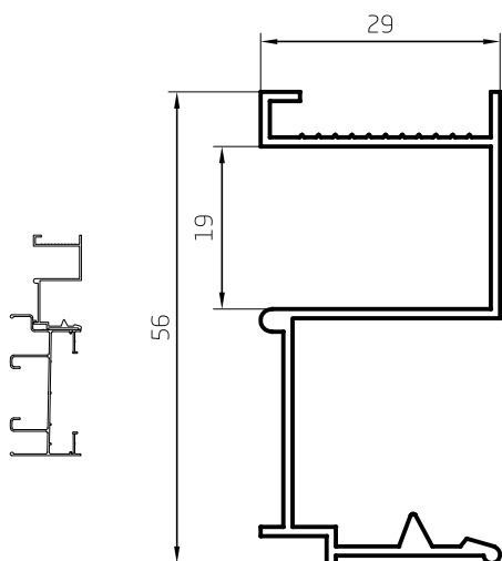
Guía Cortina de Enrollar 0,488 kg/m 00109 Barras de 6,05m 9 Barras por Paquete
