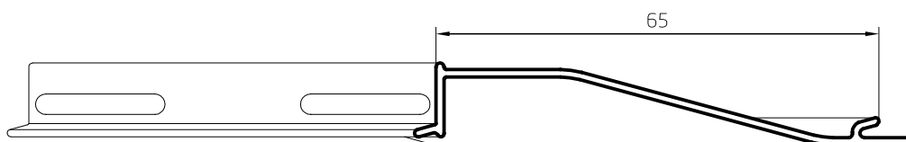
Tablilla Postigón 65mm troquelada (15 tablillas / metro lineal) 0,265 kg/m 00428 Barras de 6,05m 15 Barras por Paquete
