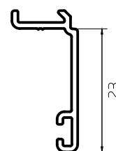
Tapajuntas 0,148 kg/m 09013 Barras de 6,05m 20 Barras por Paquete
