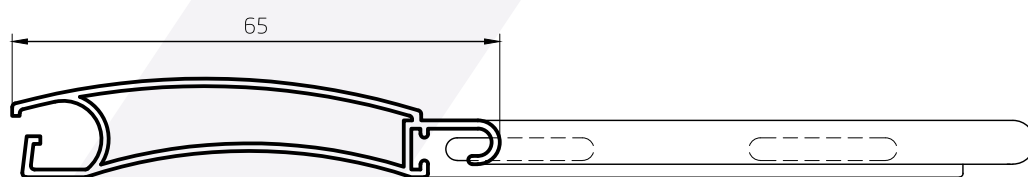
Tablilla Cortina de Enrollar troquelada 0,426 kg/m 00433 Barras de 6,05m 10 Barras por Paquete
