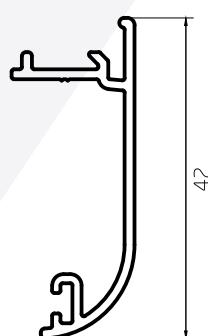
Tapajuntas Curvo 0,312 kg/m 09012 Barras de 6,05m 18 Barras por Paquete
