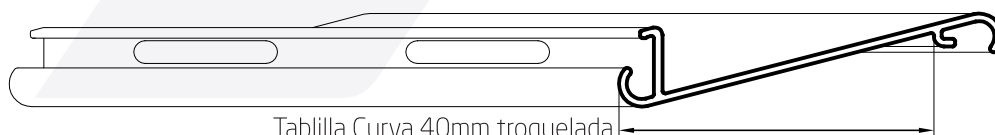
Tablilla Curva 40mm (25 tablillas / metro lineal) 0,203 kg/m 00419 Barras de 6,05m 20 Barras por Paquete
