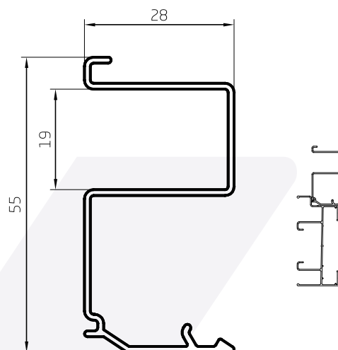
Guía Cortina de Enrollar Liviana 0,450 kg/m 00169 Barras de 6,05m 12 Barras por Paquete
