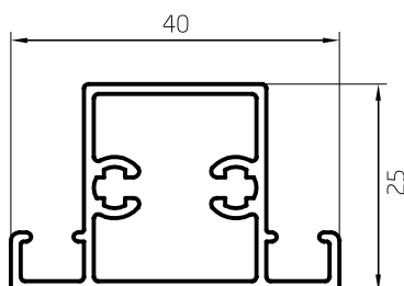
Travesaño Puerta Mosquitero 0,501 kg/m 00120 Barras de 6,05m 9 Barras por Paquete
