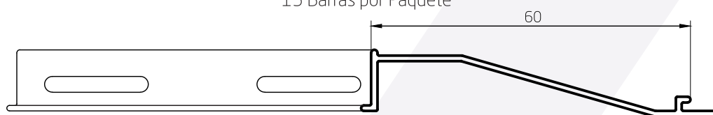
Tablilla Postigón 60mm troquelada (15 tablillas / metro lineal) 0,248 kg/m 00430 Barras de 6,05m 15 Barras por Paquete
