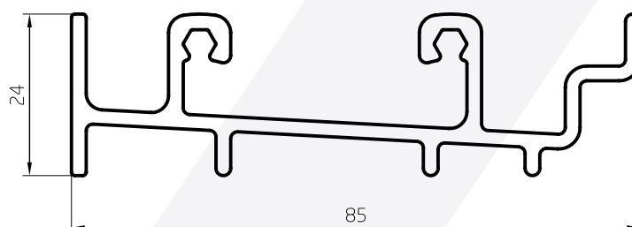
Marco Transitable 24mm 1,202 kg/m 00130 Barras de 6,05m 4 Barras por Paquete
