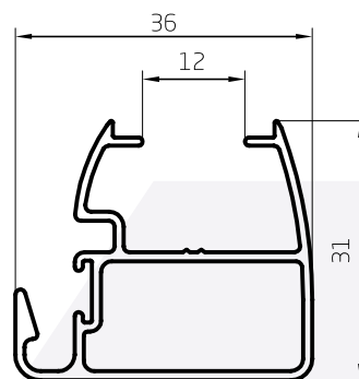
Parante Central Curves 0,449 kg/m 00174 Barras de 6,05m 12 Barras por Paquete
