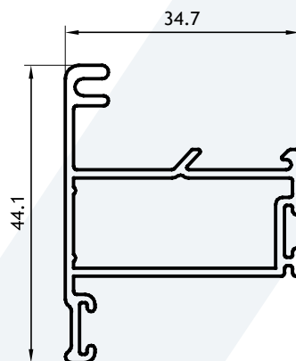
Hoja Ventiluz 0,537 Kg/m 00185 Barras de 6.05m 6 Barras por Paquete
