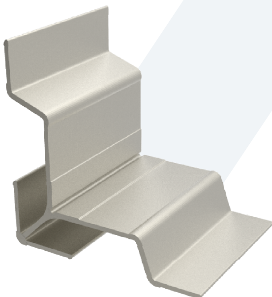
70604 Escuadra de aluminio 13mm para premarco 147 de 45.5mm x 100 unidades
