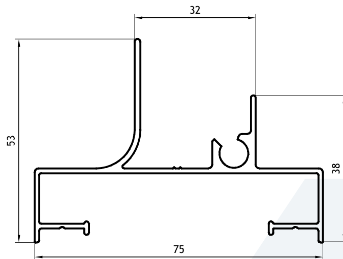
Marco Ventiluz 0,779 Kg/m 00184 Barras de 6.05m 4 Barras por Paquete
