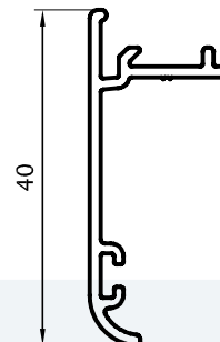
Tapajuntas 0,251 kg/m 09011 Barras de 6.05m 18 Barras por Paquete
