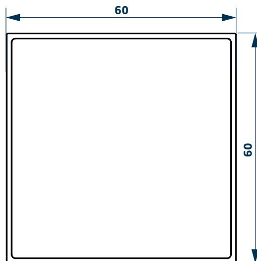
Caño cuadrado 60x60x1.3mm 01107 0,842 kg/m Barras de 6,05m 4 Barras por Paquete
