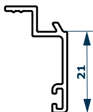
Tapajuntas 02810 0,175 kg/m Barras de 6,20m 12 Barras por Paquete
