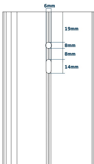
Mecanizado de marco para escuadra Cód. 70383
