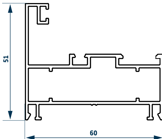
Marco de abrir Patagonia Plus vidrio simple
