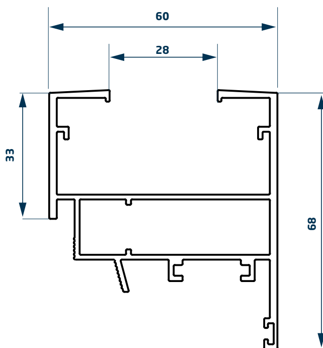
Hoja de abrir Patagonia dvh Plus
