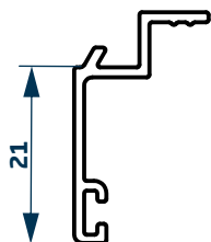
Tapajunta recto 20mm 02810 0,175 kg/m Barras de 6,20m 12 Barras por Paquete
