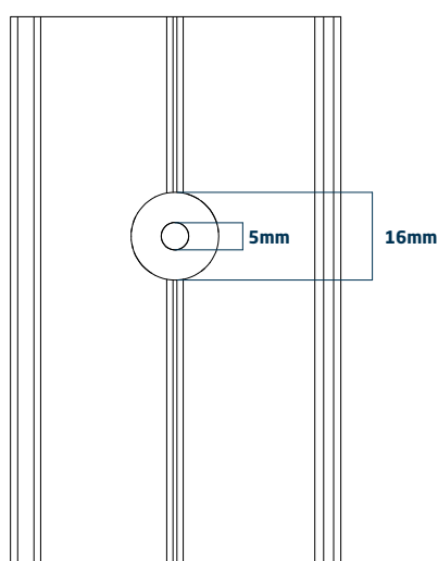
Mecanizado para taco regulador Cód. 03442
