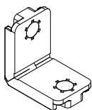
Escuadra a tracción Ø 8 marco de abrir Patagonia Plus (E-83) Cód. 70383
