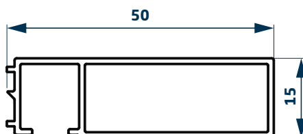
Premarco 50mm 03415 0,411 kg/m Barras de 6,20m 10 Barras por Paquete
