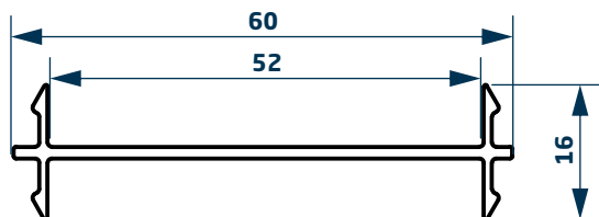
Unión 180° plus 03414 0,322 kg/m Barras de 6,20m 6 Barras por Paquete
