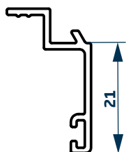
Tapajuntas recto 20mm 02810 0,175 kg/m Barras de 6,20m 12 Barras por Paquete
