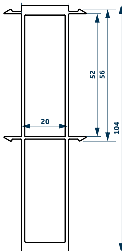
Unión 180° plus reforzada 03417 1,326 kg/m Barras de 6,20m Barras por Paquete
