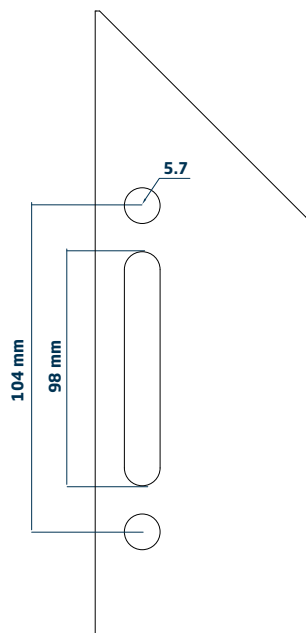
Mecanizado de hoja para falleba Cód. 03441
