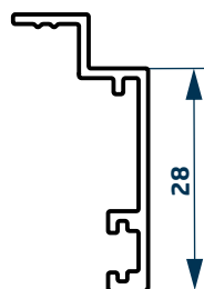
Tapajuntas 28mm 03411 0,215 kg/m Barras de 6,20m 10 Barras por Paquete
