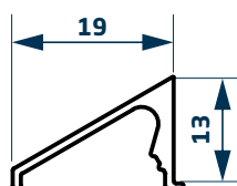
Perfil botaguas 03428 0,137 kg/m Barras de 6,20m 12 Barras por Paquete
