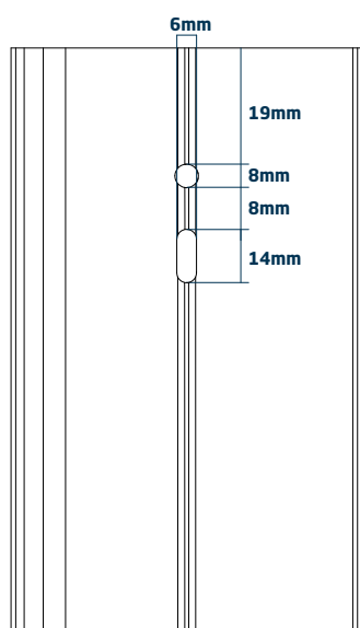
Mecanizado de marco para escuadra Cód. 03442
